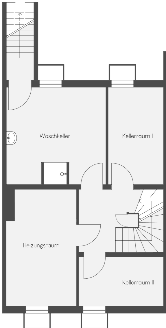
Grundriss Kellergeschoss
