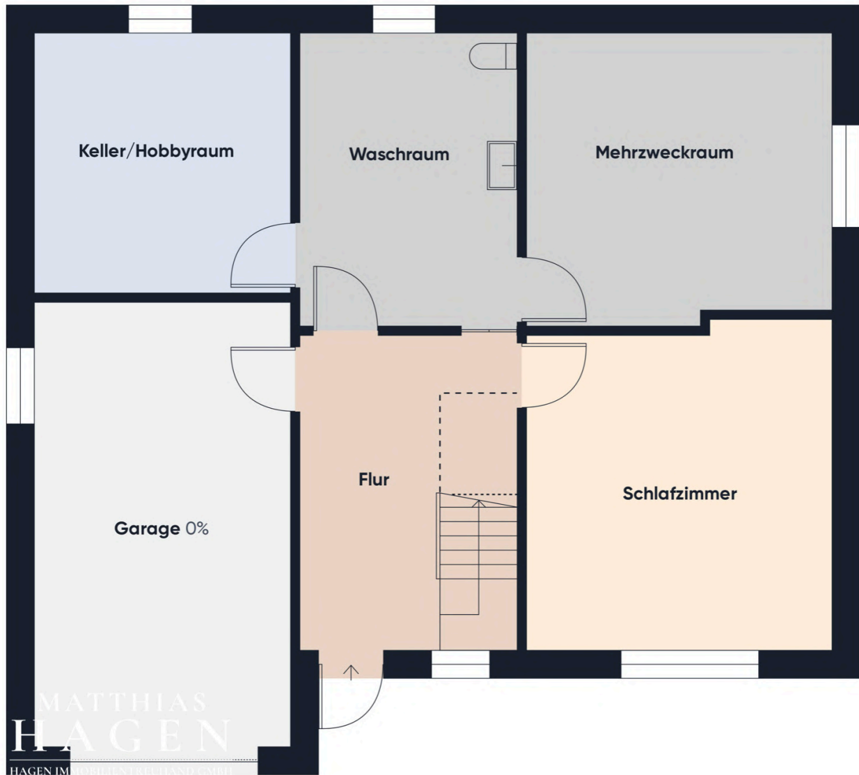
Grundriss EG ohne Maßstab
