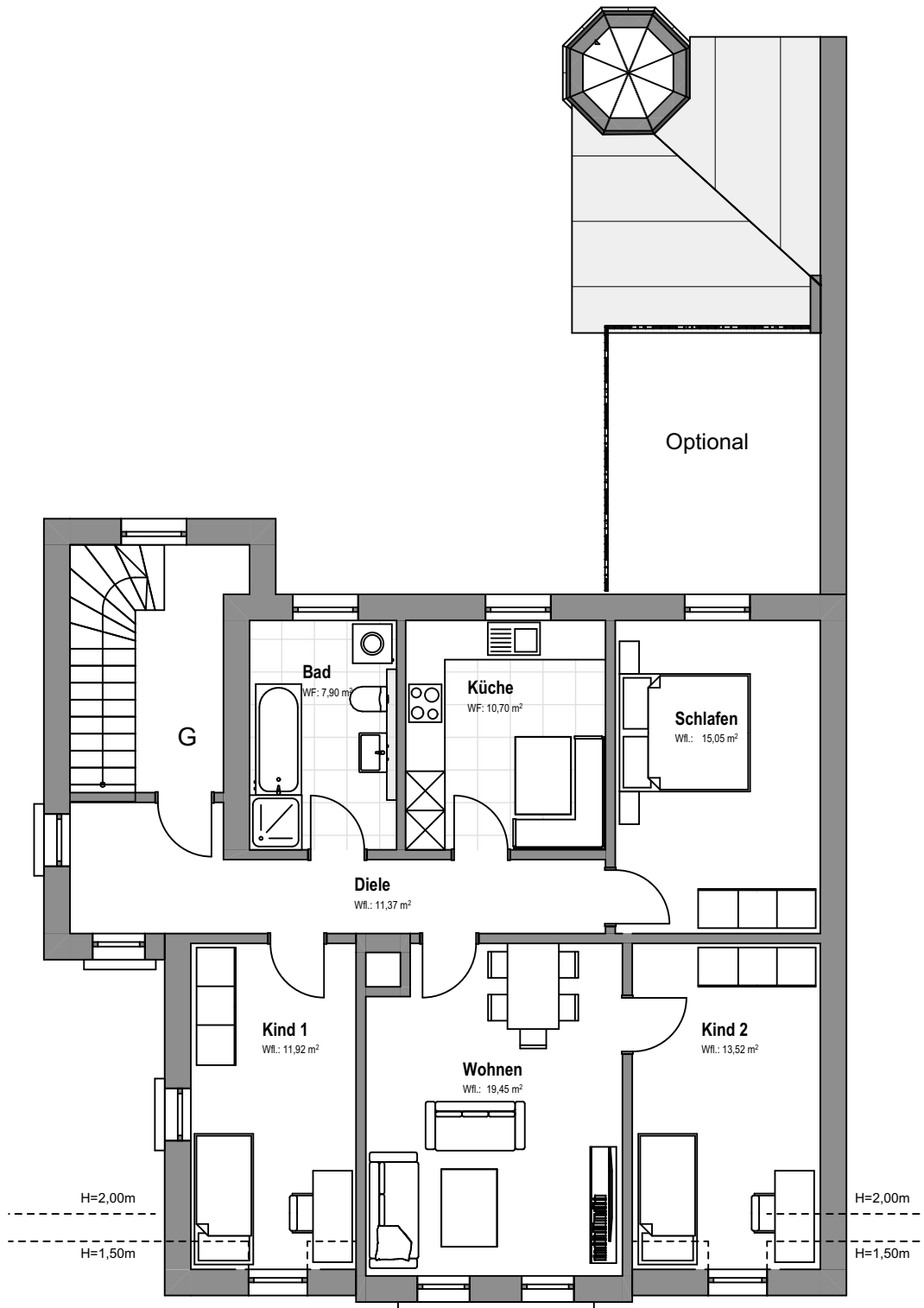
Grundriss DG
