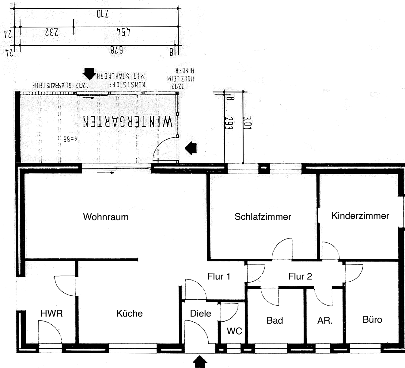
Grundriss Wintergarten 1 : 100
