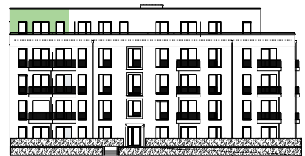
ANSICHT SÜD
