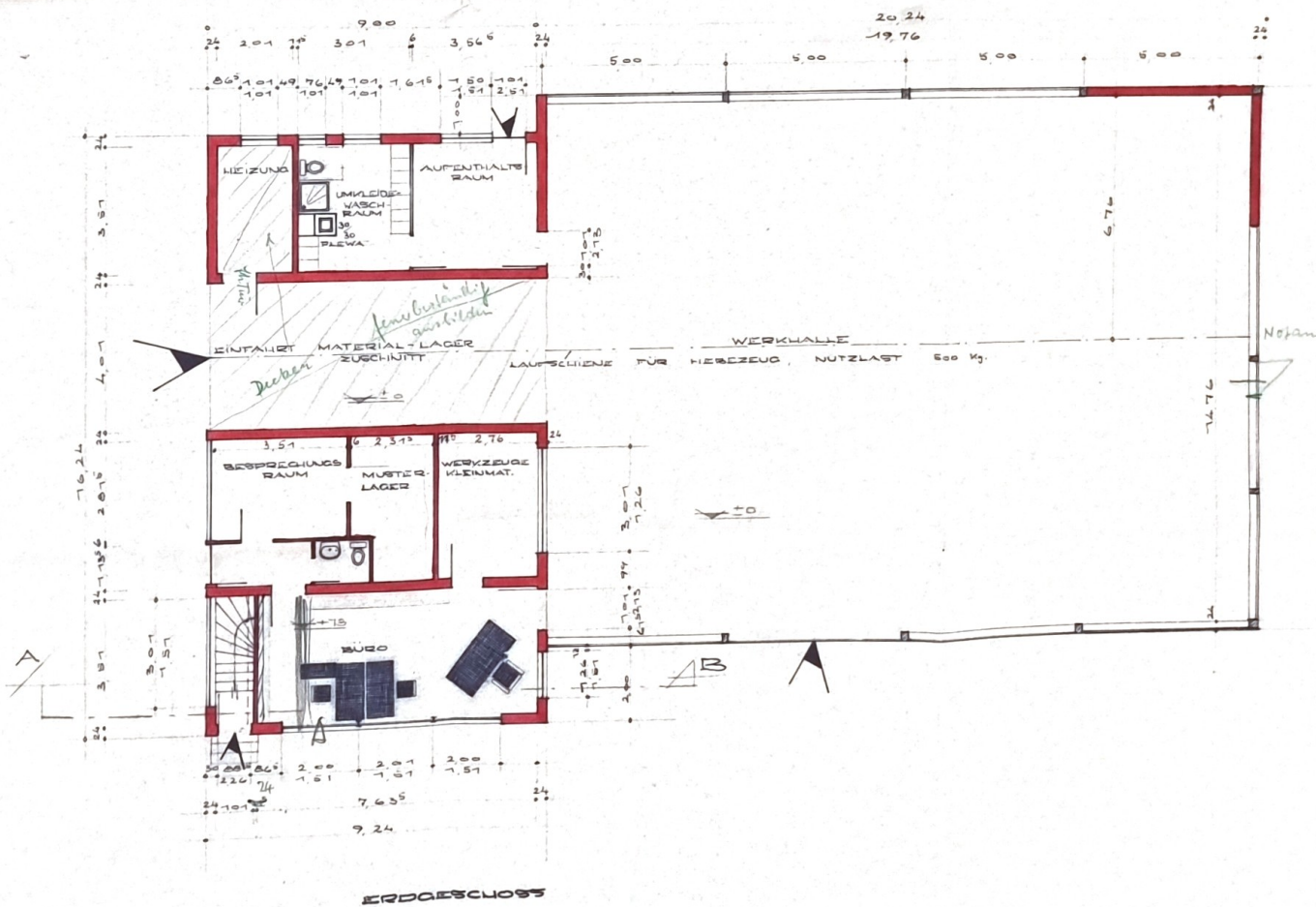
ERDGESCHOSS
