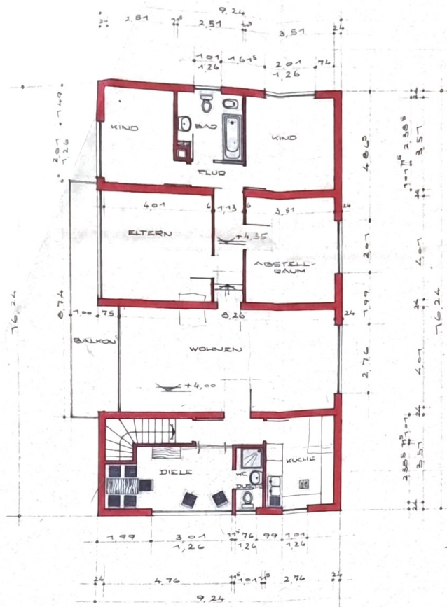
OBERGESCHOSS
