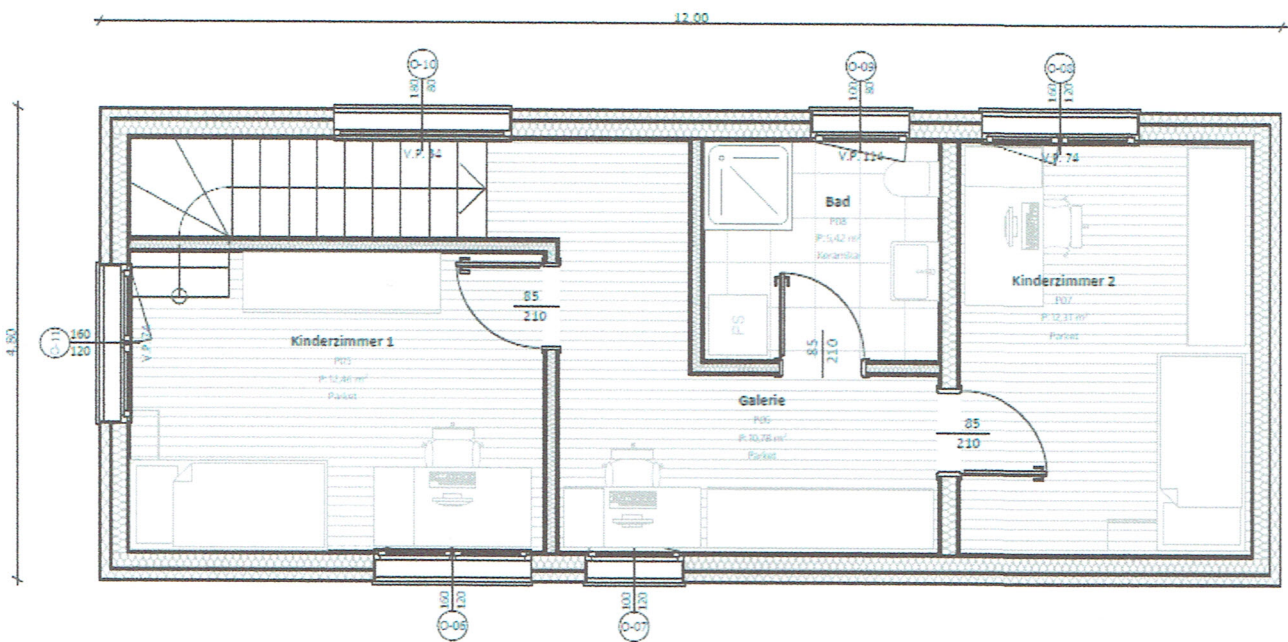
Grundriss Etage
