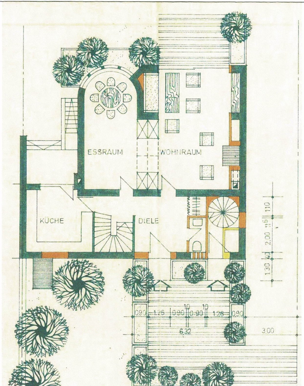
GRUNDRISS ERDGESCHOSS
