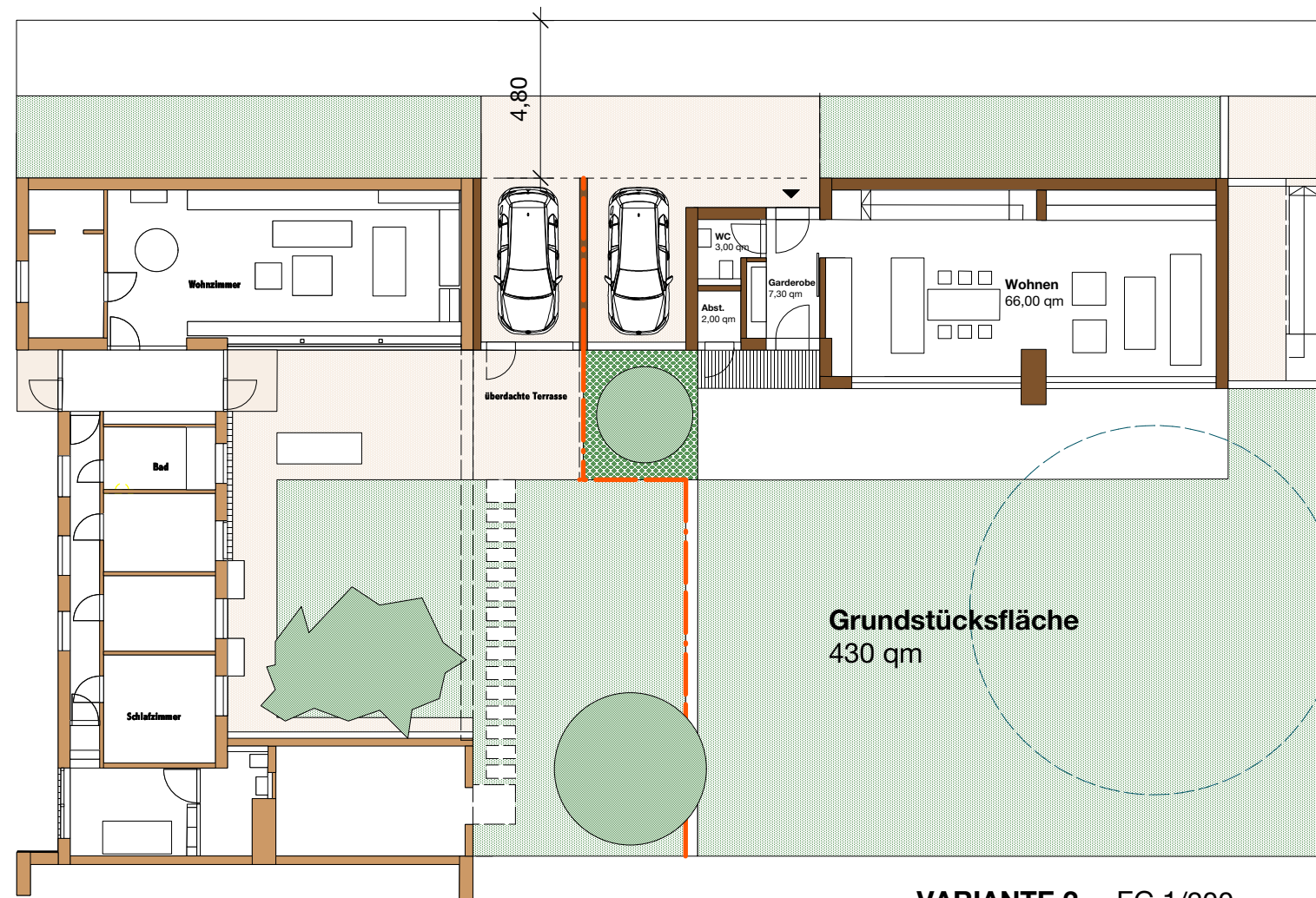
VARIANTE 2 EG 1/200
