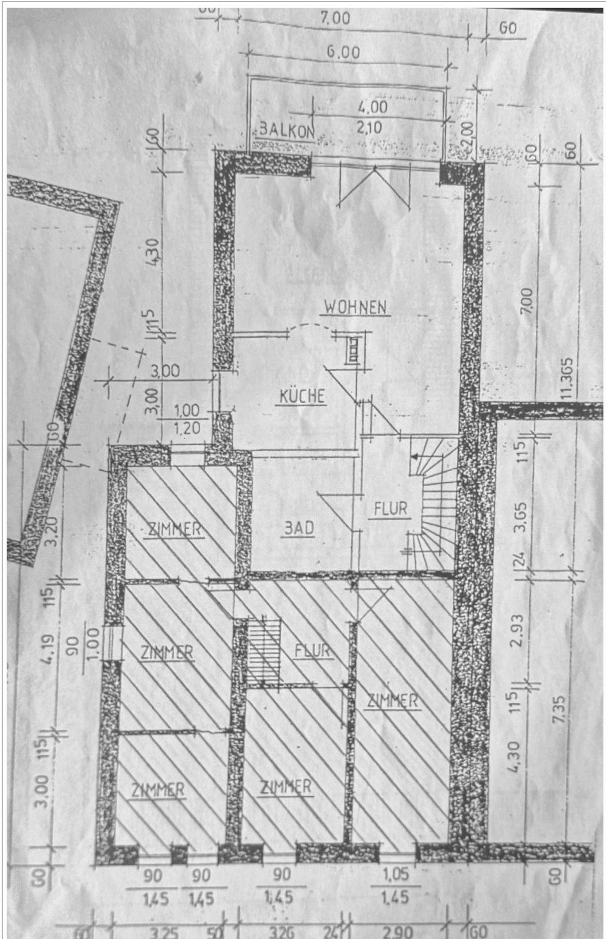
GRUNDRISS OBERGESCHOSS
