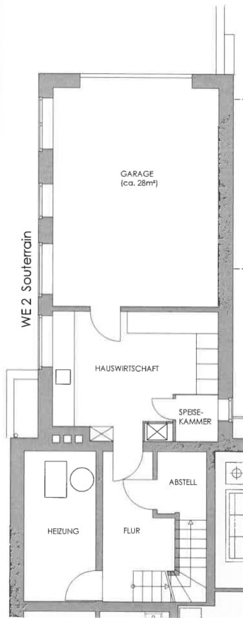
Souterrain
