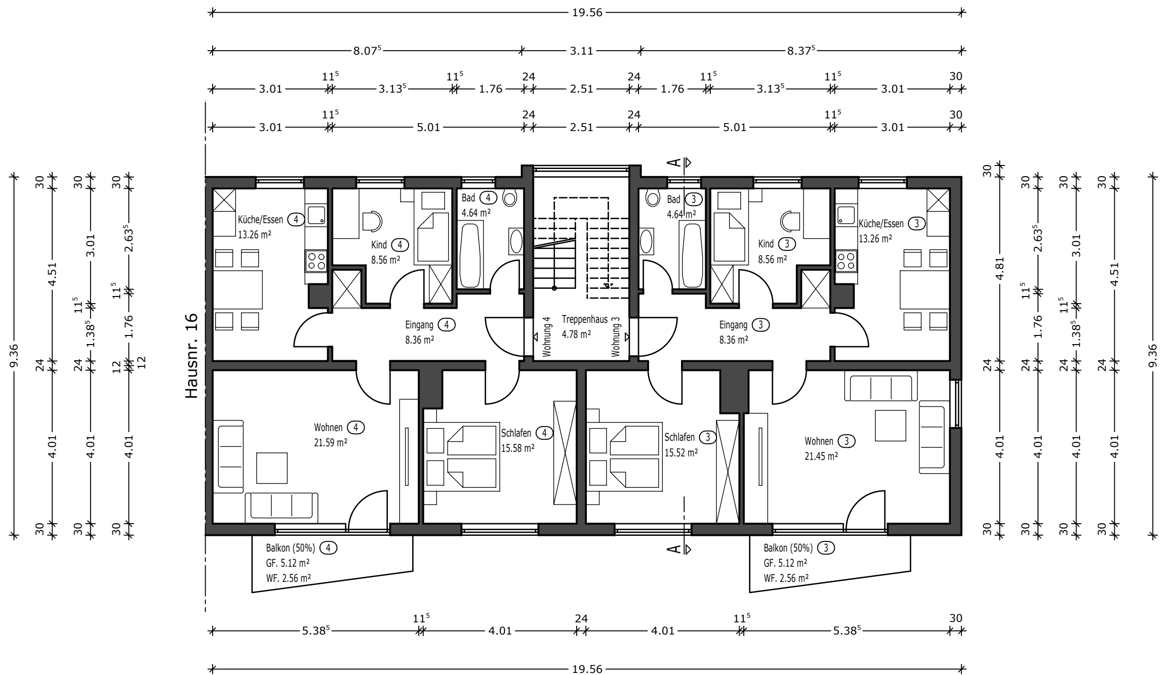
Grundriss 1.Obergeschoss (Hausnummer 14)
