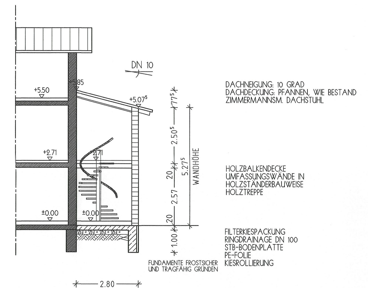
SCHNITT B-B
