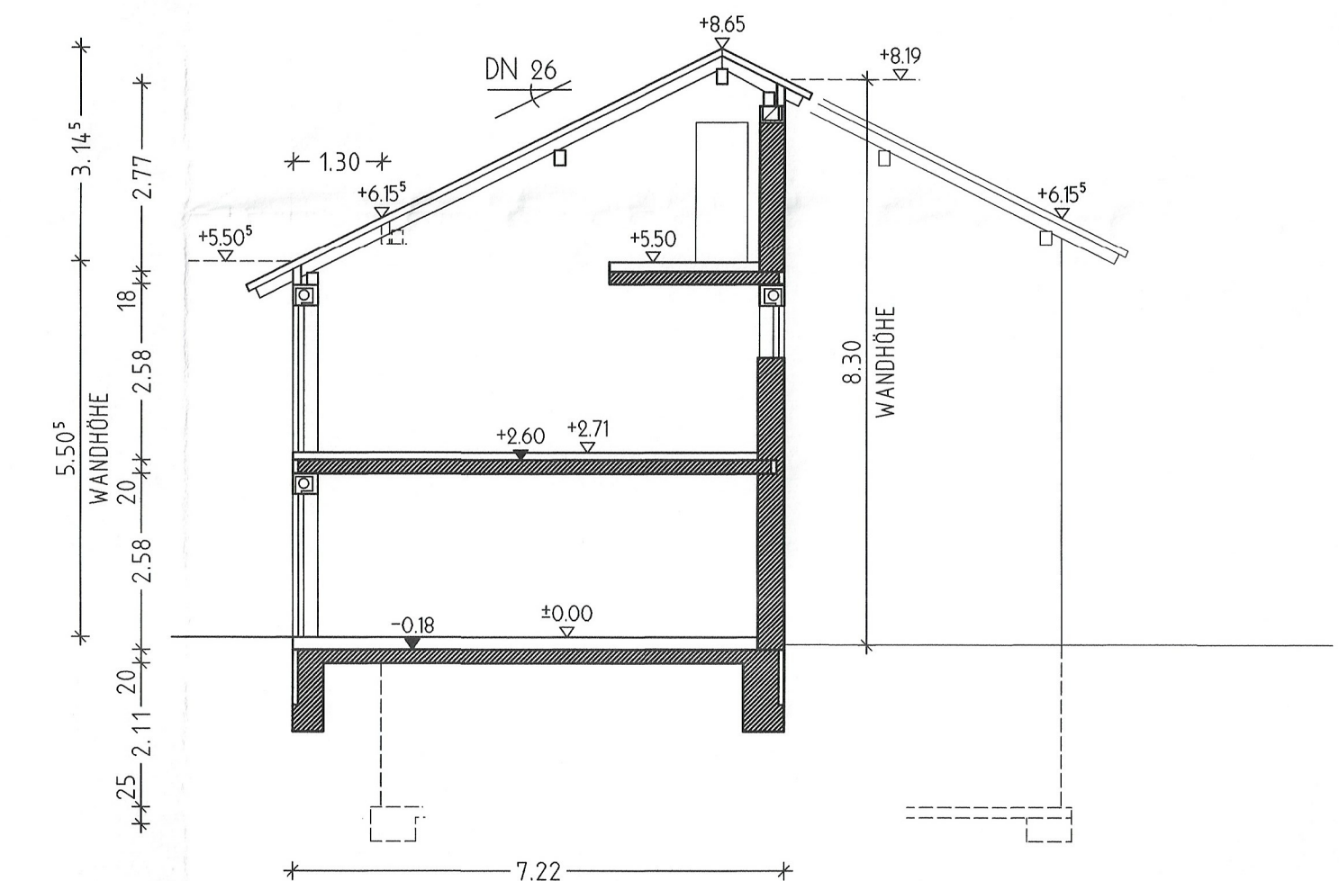
SCHNITT A-A
