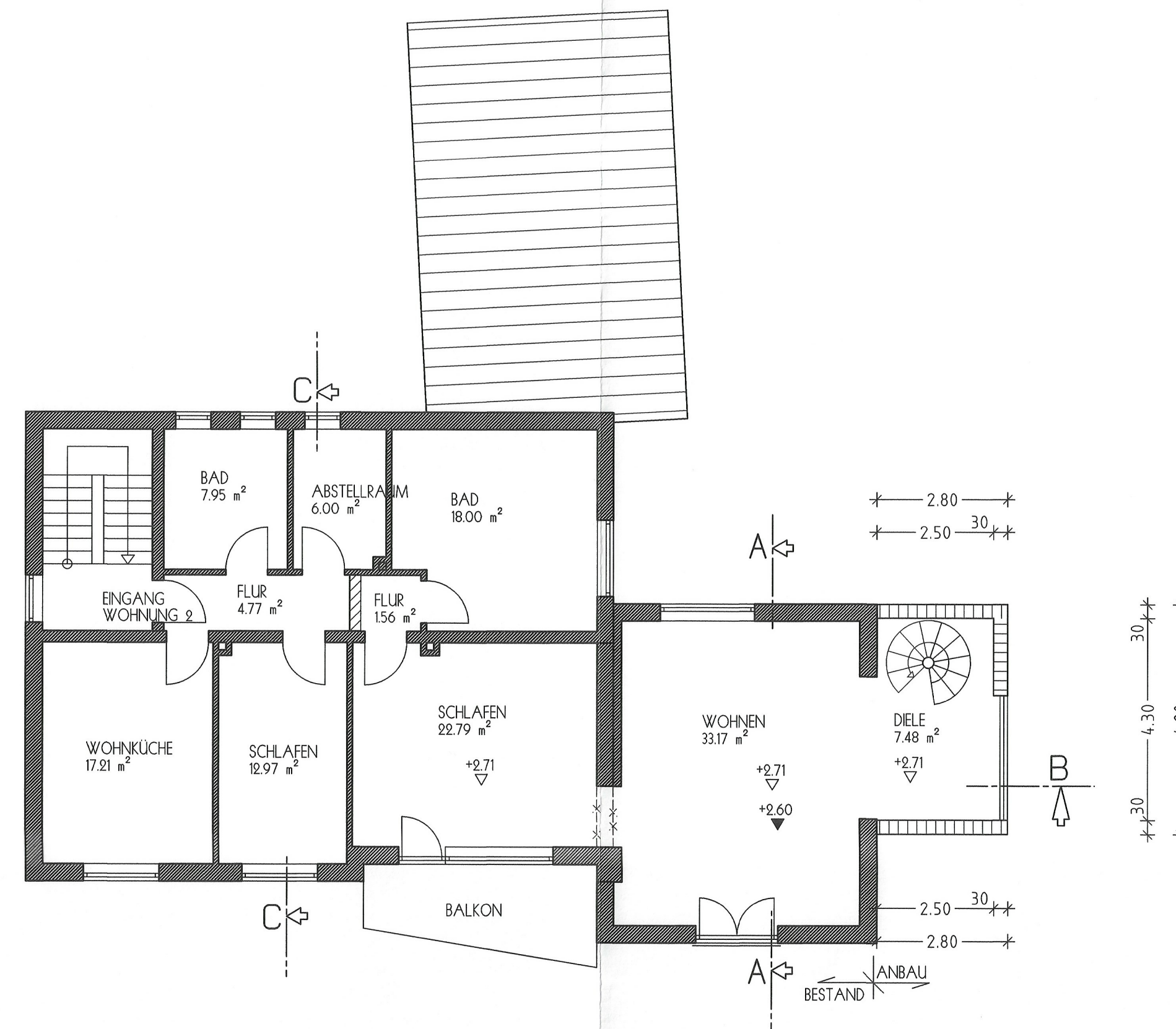
OBERGESCHOSS
