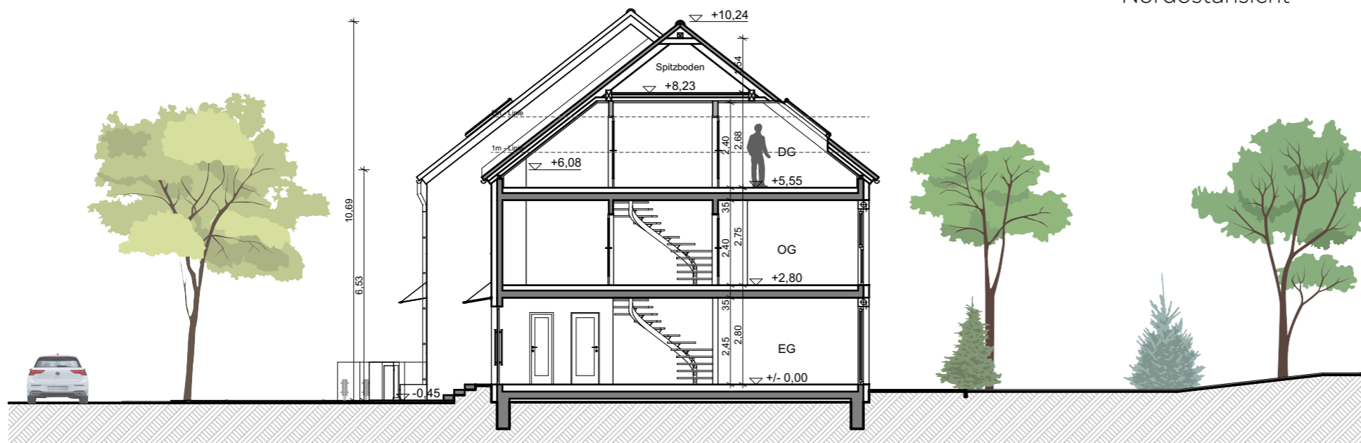
Schnitt - A
