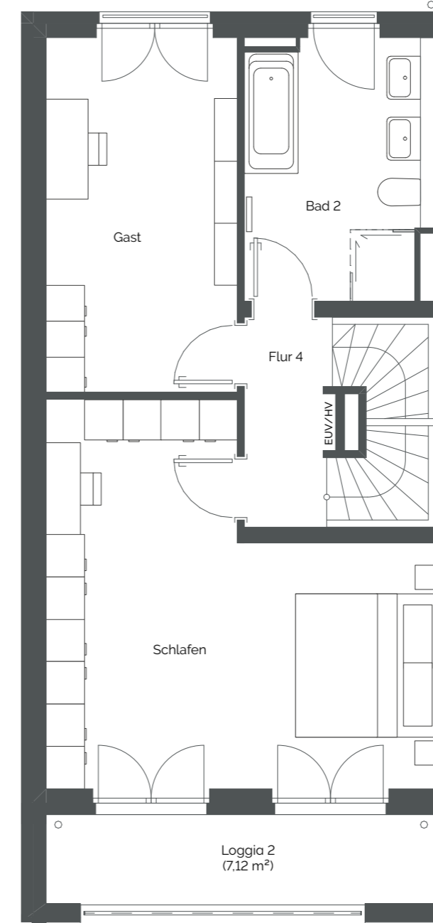
2. Obergeschoss
