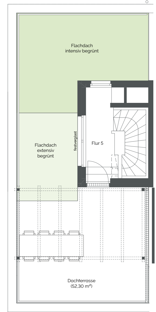
Dachgeschoss
