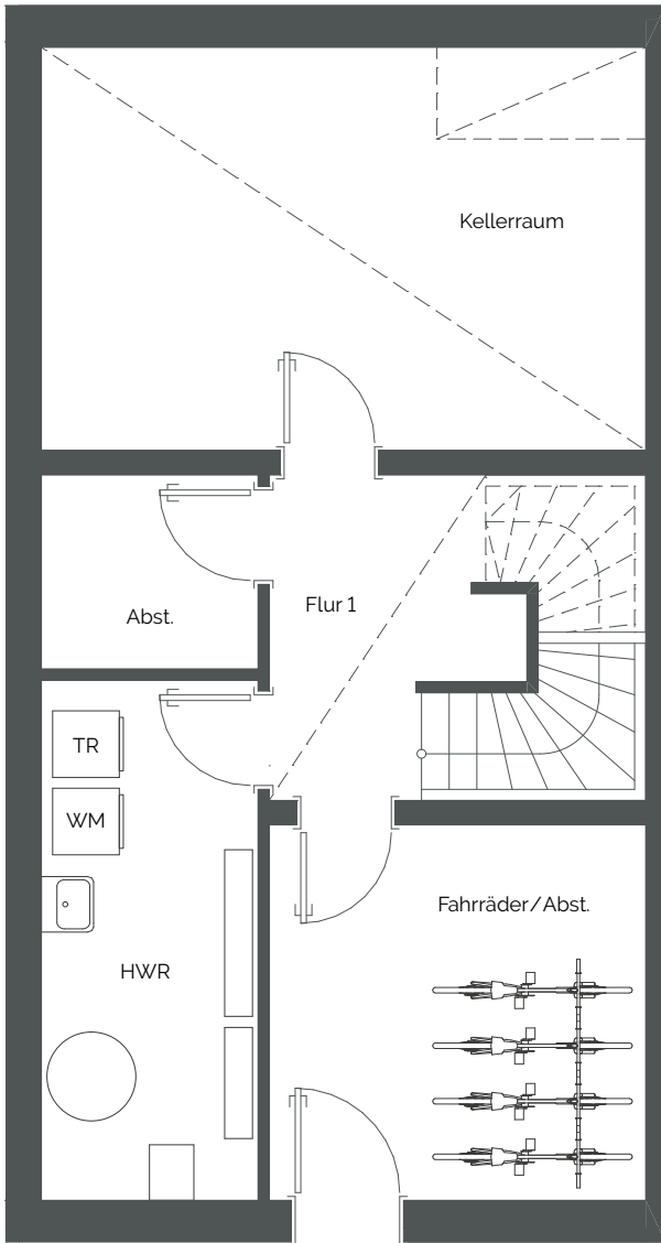
Kellergeschoss
