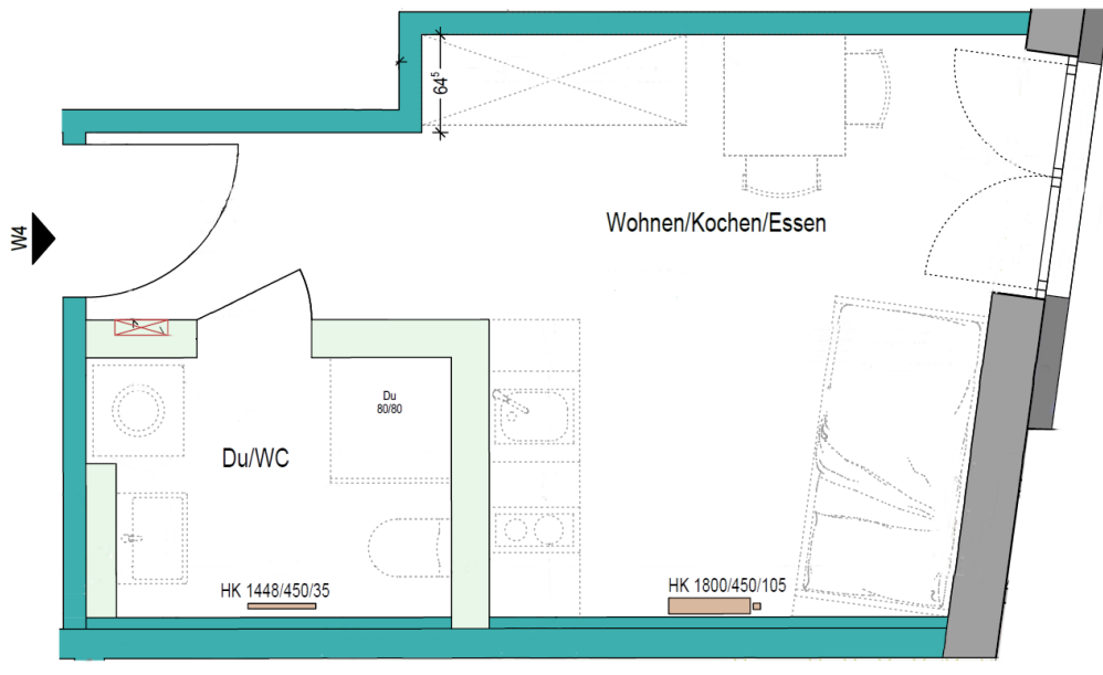
Grundriss Apartment Nr. 4 (baugleich mit Nr. 8)
