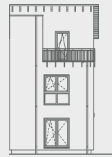
Ansicht Hinten
