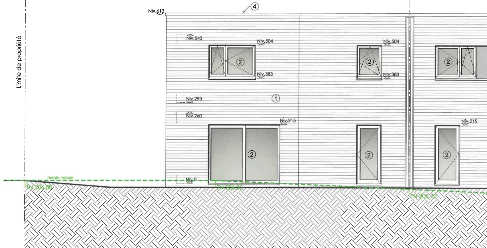
Façade Nord - coupe dans terrain (Ech. 1%)
