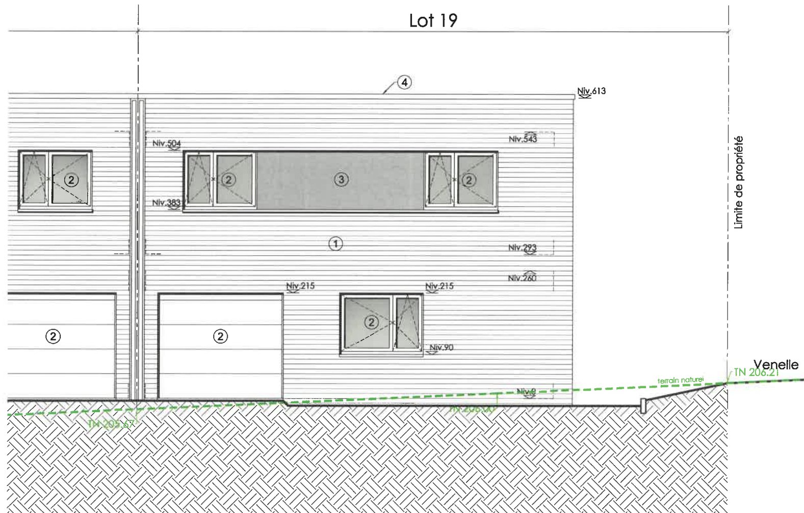
Façade Sud - lot 19 - coupe dans terrain (Ech. 1%)
