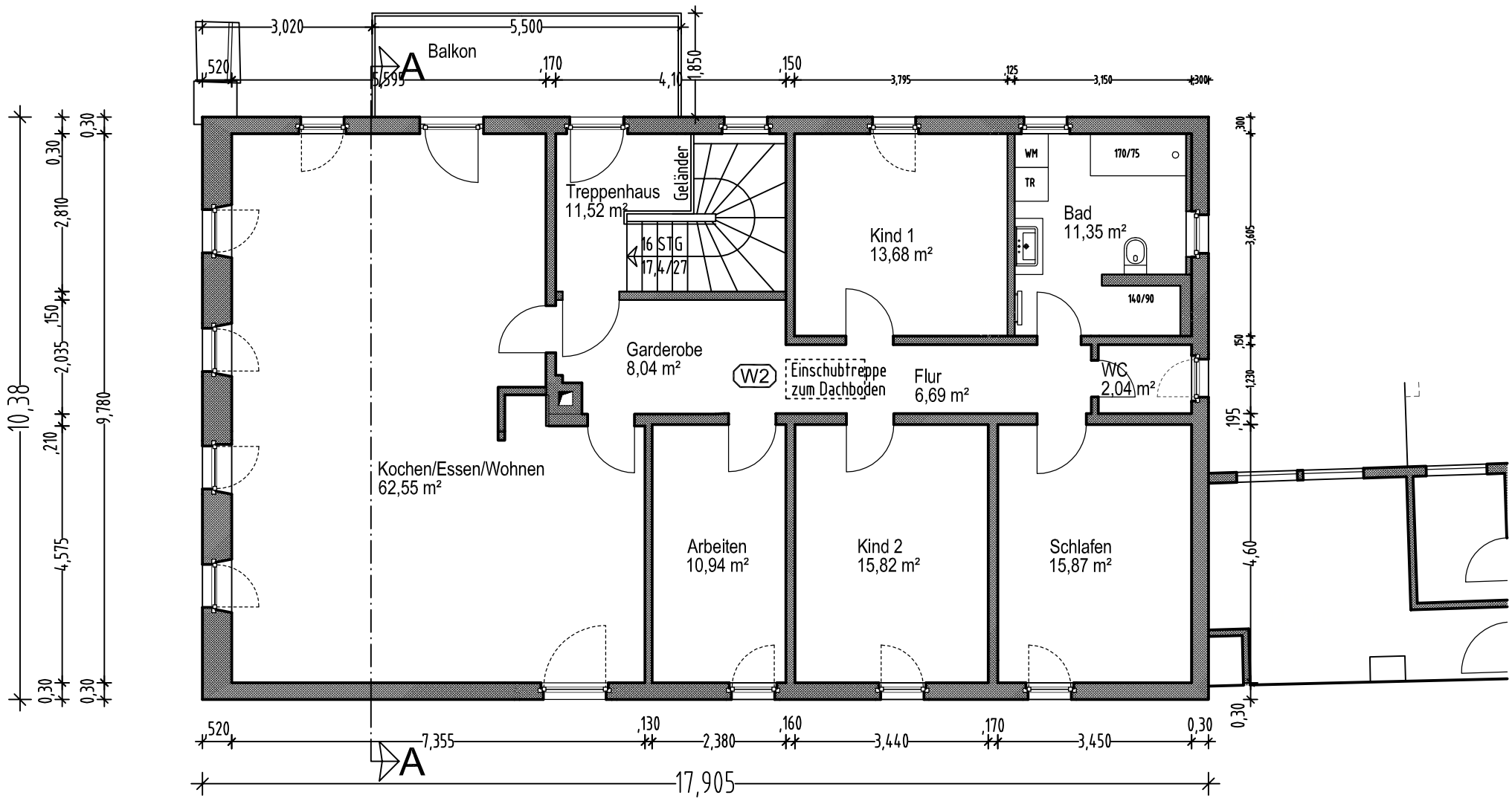
Grundriss OG M. 1 : 100
