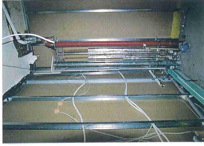
Vorbereitung des Heizraumes für die Zentralheizung mit zentraler Wasserversorgung ( Zusatzleistung )
