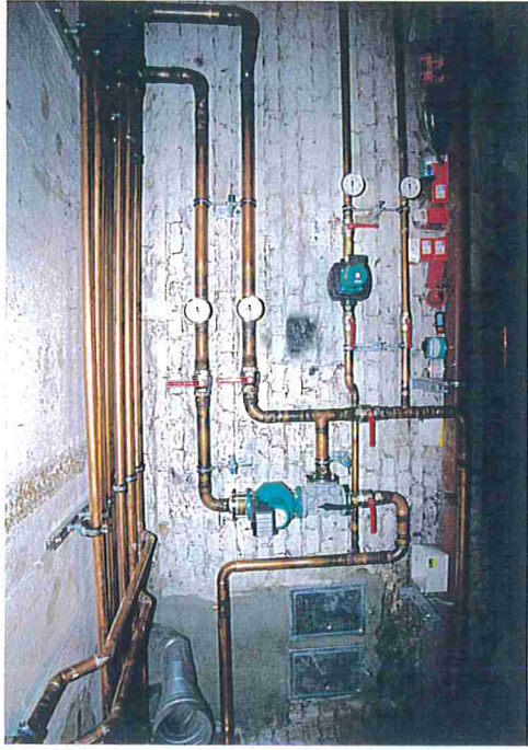
Vorbereitung des Heizraumes für die Zentralheizung mit zentraler Wasserversorgung ( Zusatzleistung )
