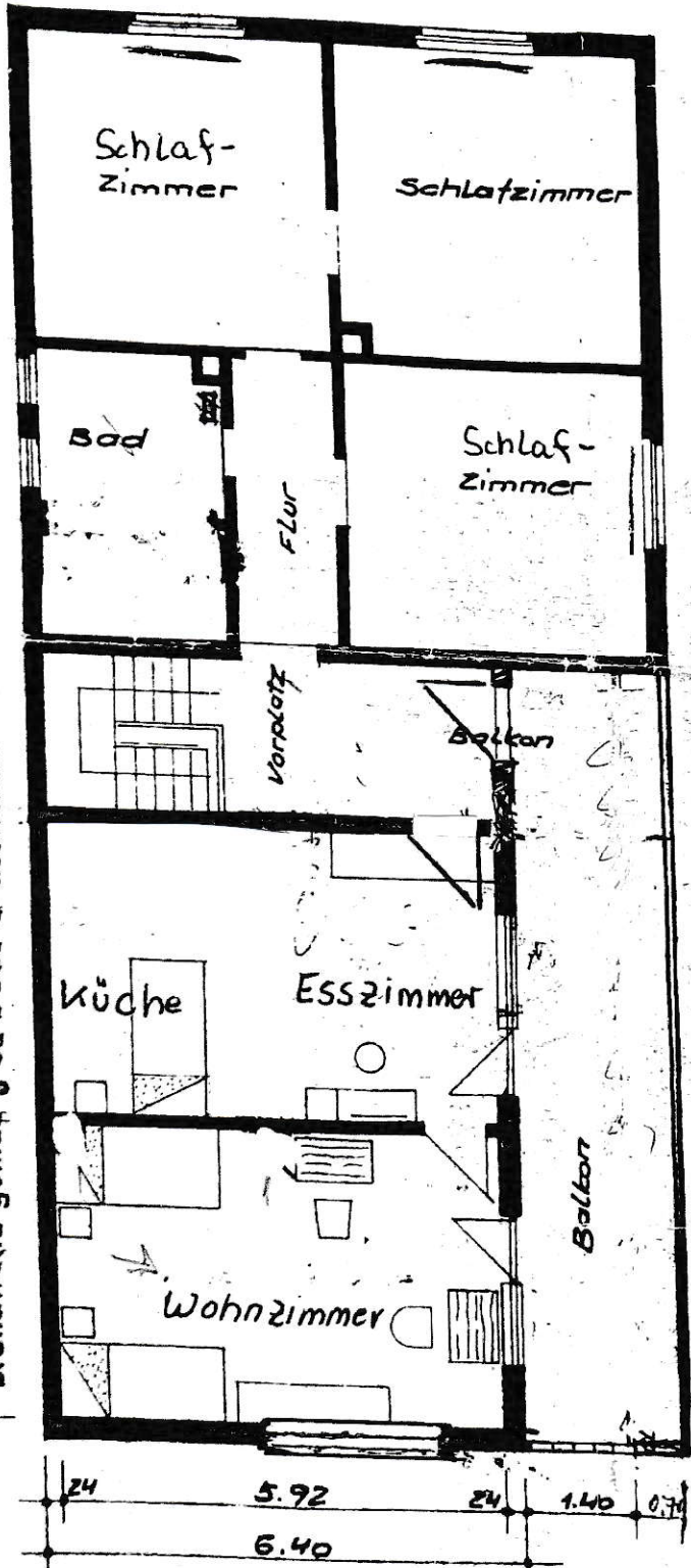
Obergeschoss MST. 1:100
