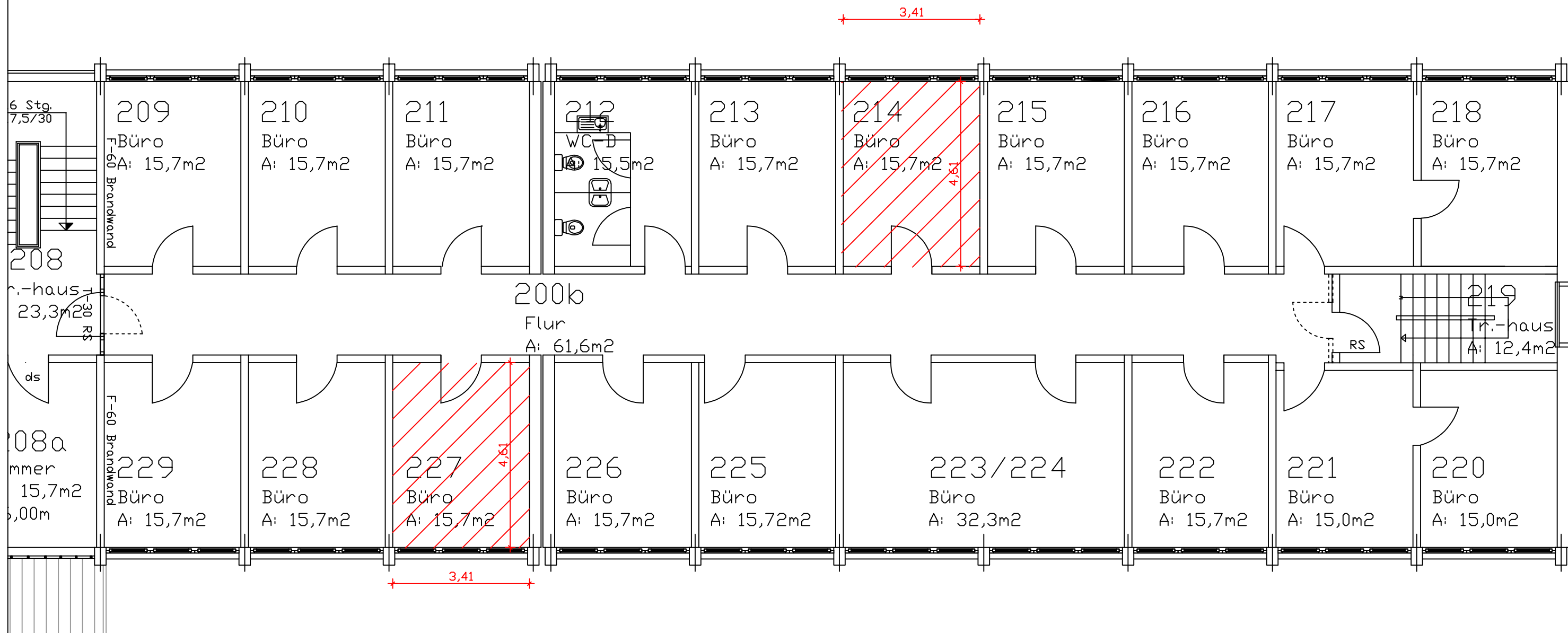
Teilgrundriss M 1:100
