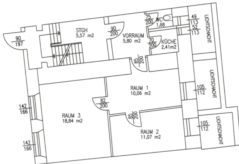
1. OBERGESCHOSS NORD - BESTAND M 1:100
