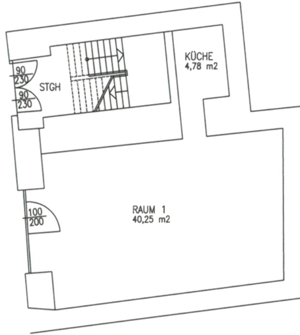
ERDGESCHOSS NORD - BESTAND M 1:100
