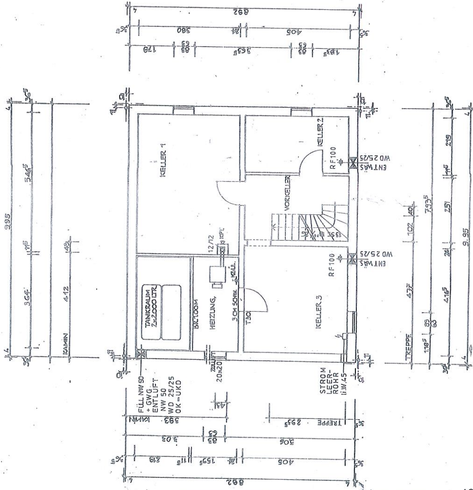
KELLERGESCHOSS
