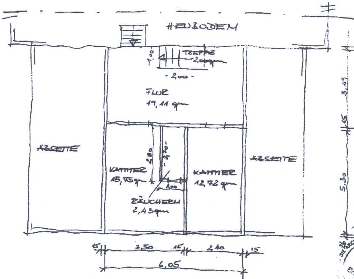
2. OBERGESCHOSS
