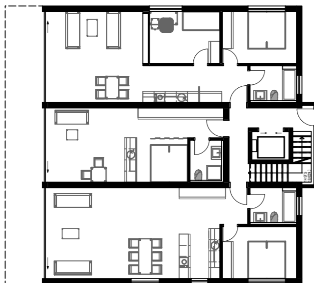
Wohnung 3 68m 2
