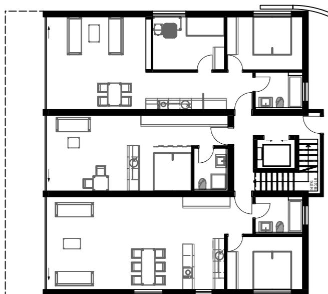
Wohnung 3 68m 2
