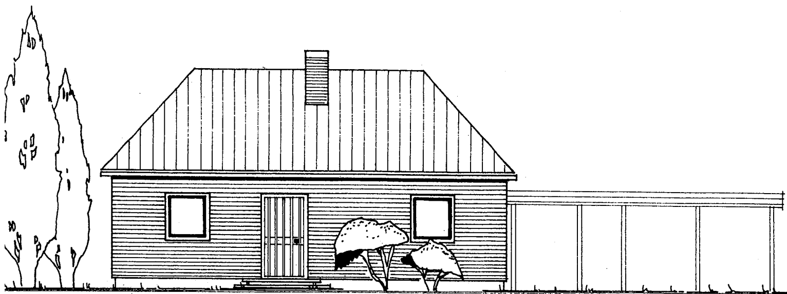
von osten
