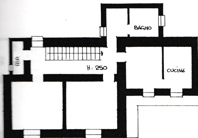
PLANIMETRIA SECONDO PIANO
