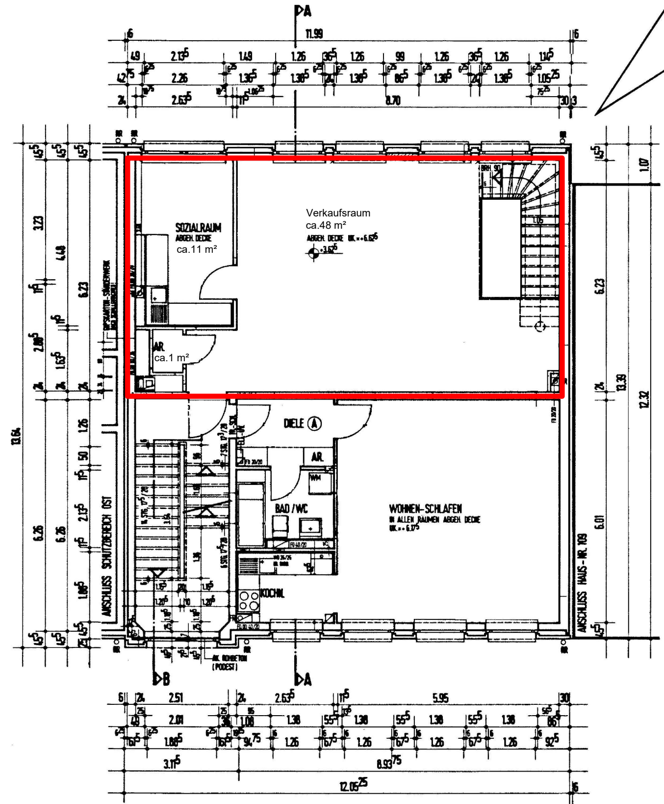
1. Obergeschoss
