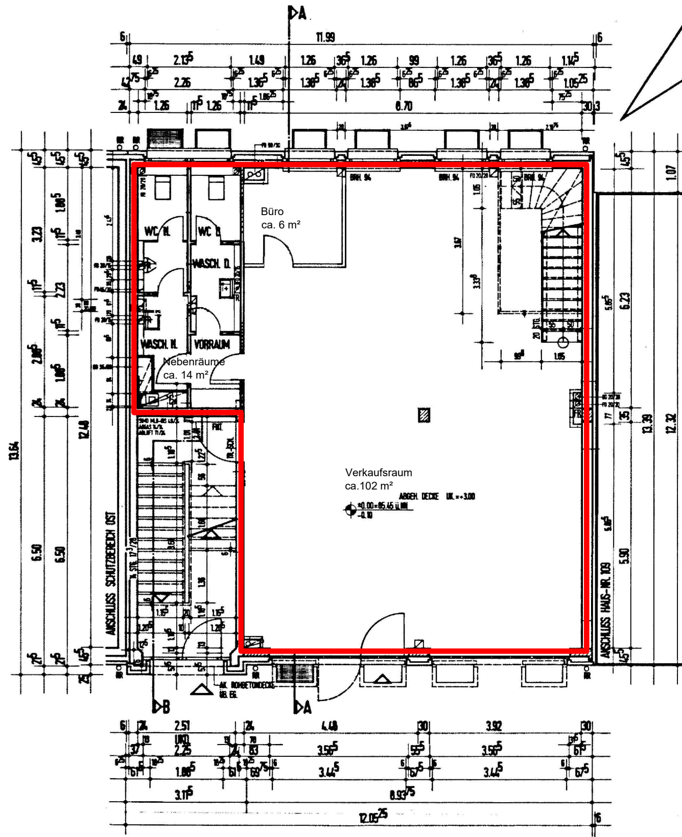
Erdgeschoss
