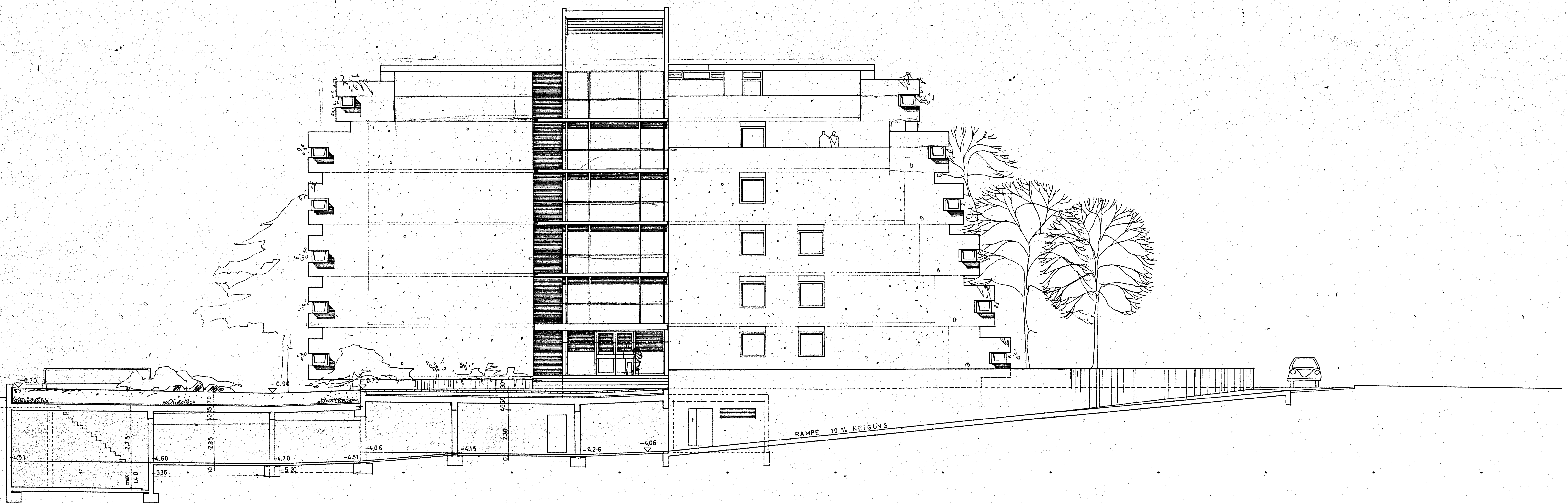
ANSICHT NORDEN + SCHNITT C-C
