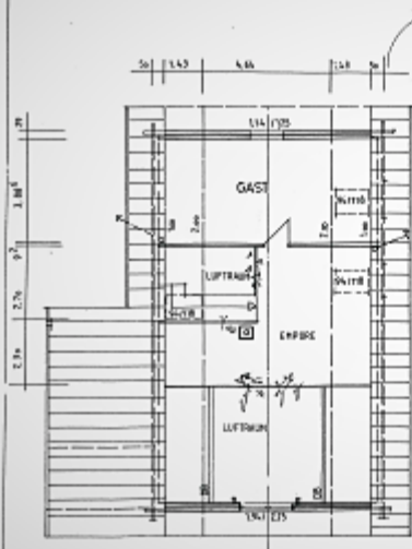
DACHGESCHÖSS M 1:100
