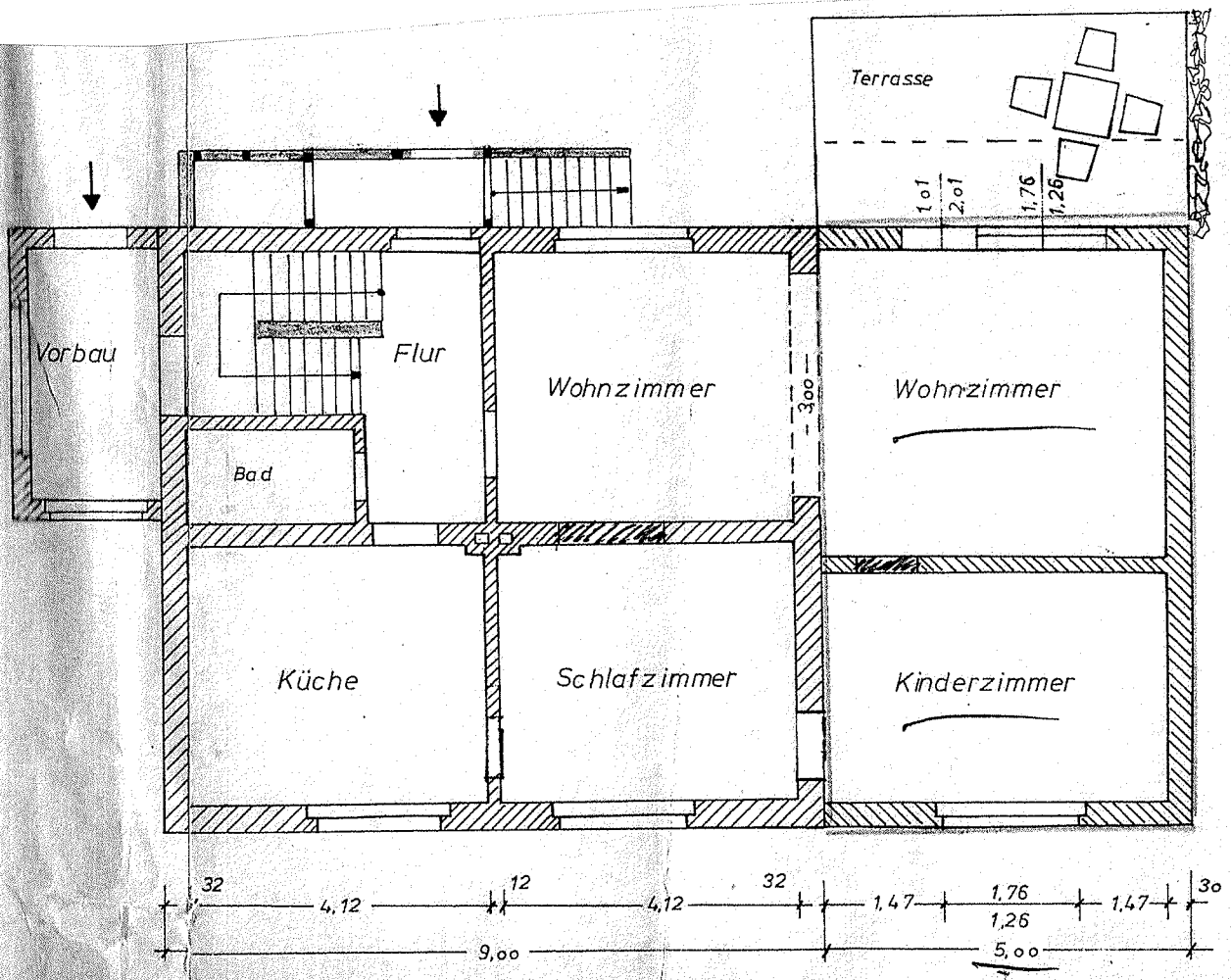
Erdgeschoß
