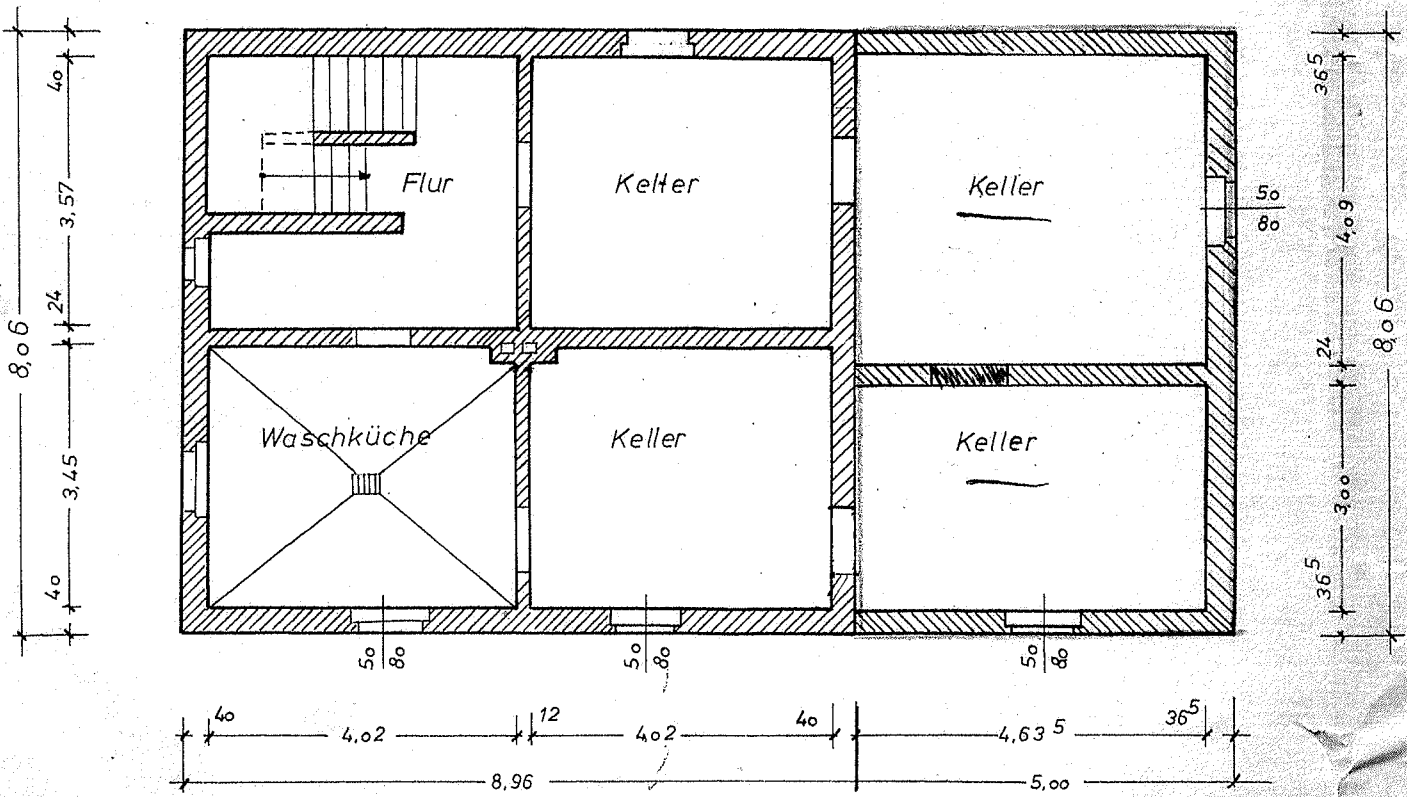
Kellergeschoß
