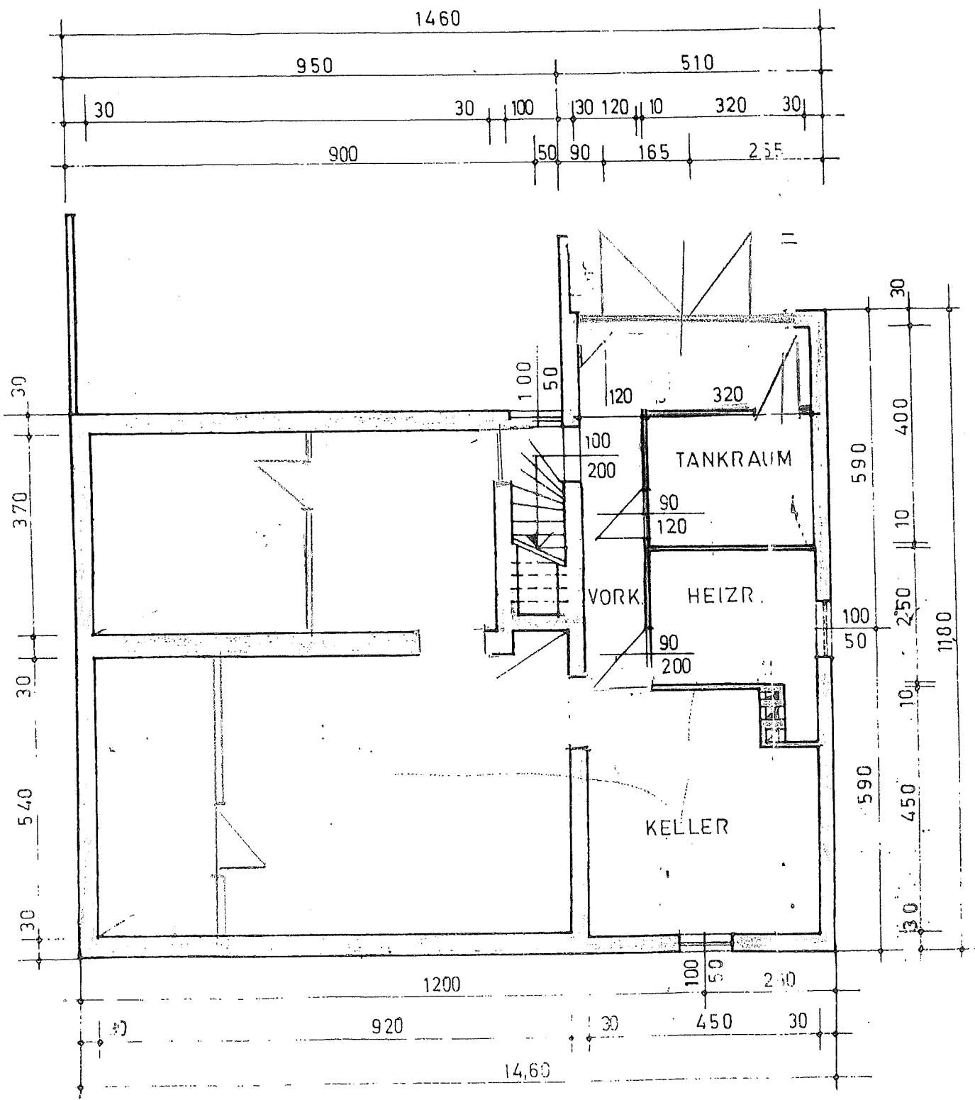
KELLERGESCHOSS
