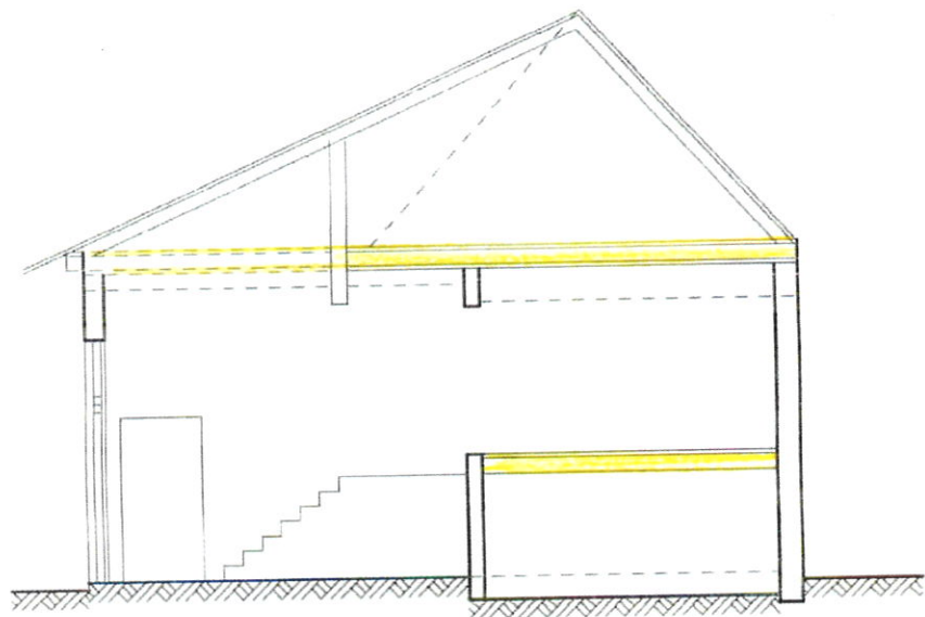
SCHNITT A-A - VORHANDEN
