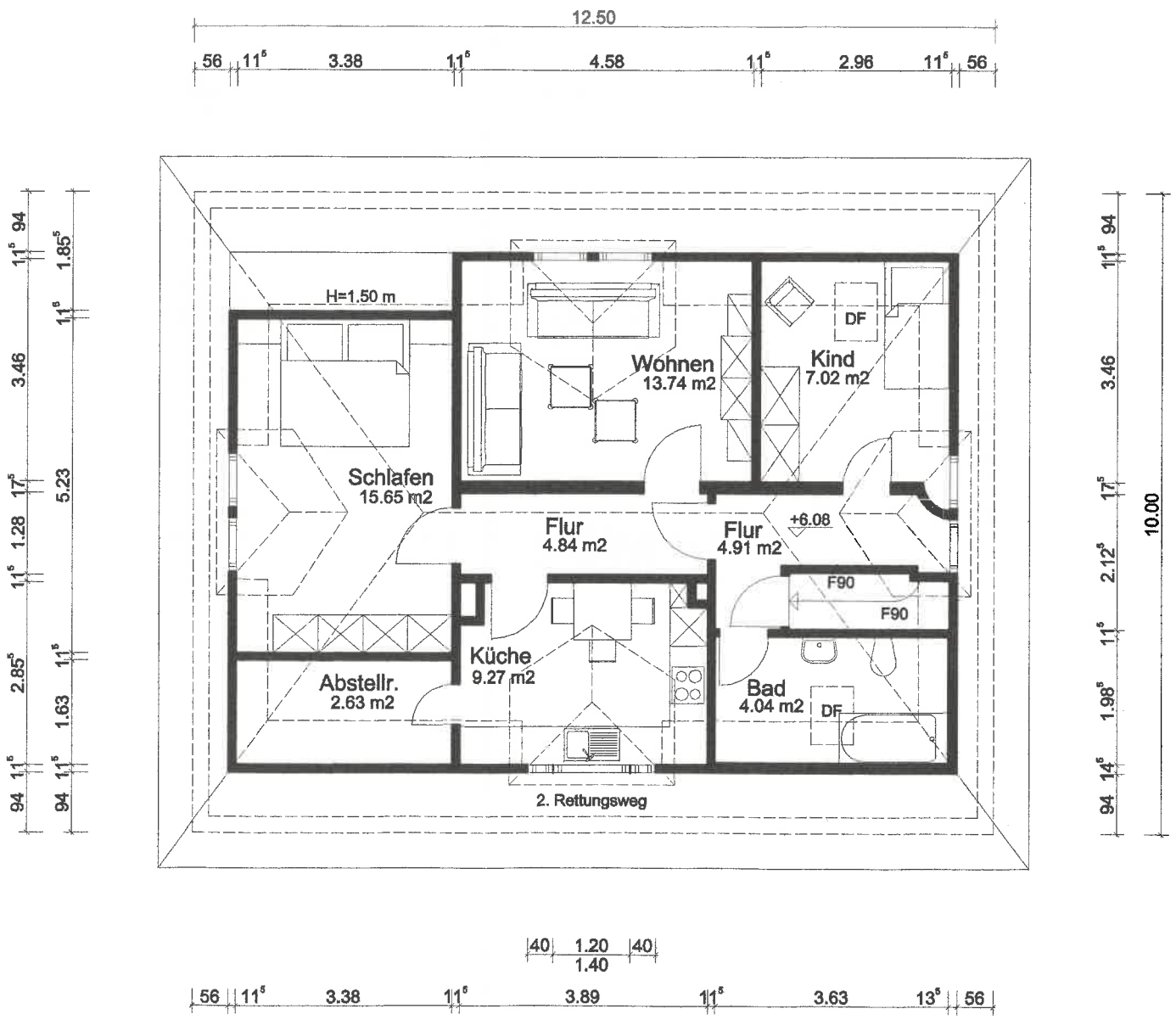
Grundriss Dachgeschoss
