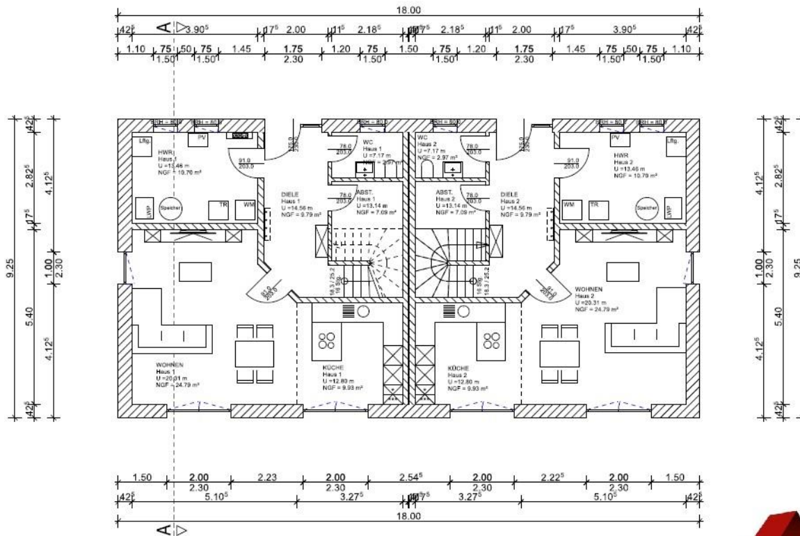
Grundriss Erdgeschoss
