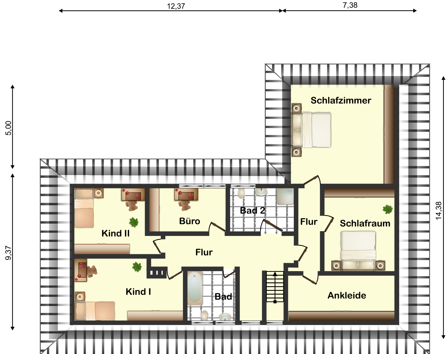
Dachgeschoss
