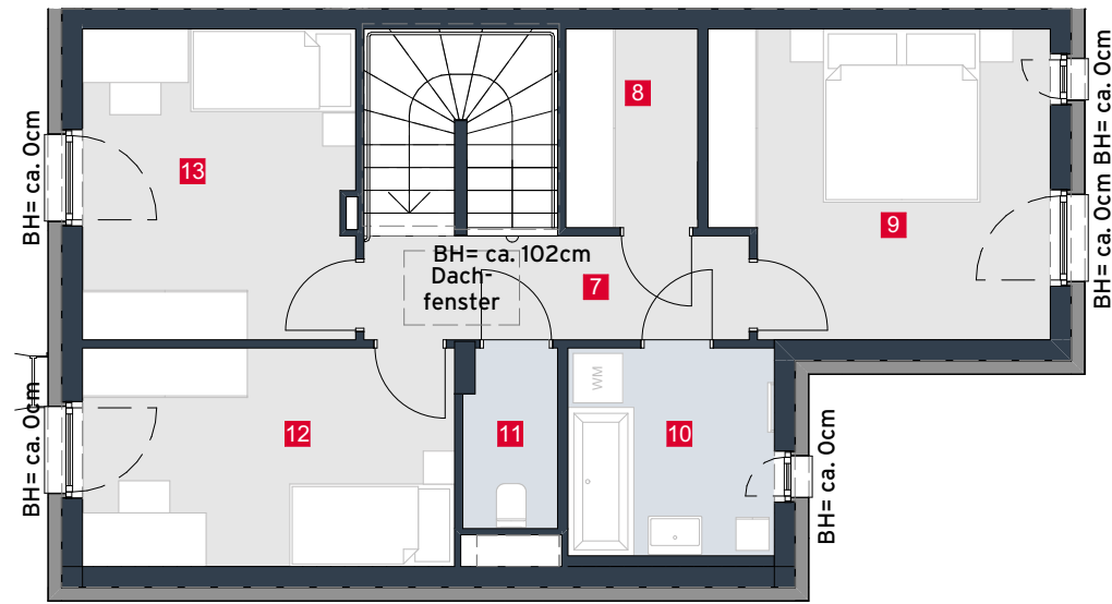
1. Obergeschoss
