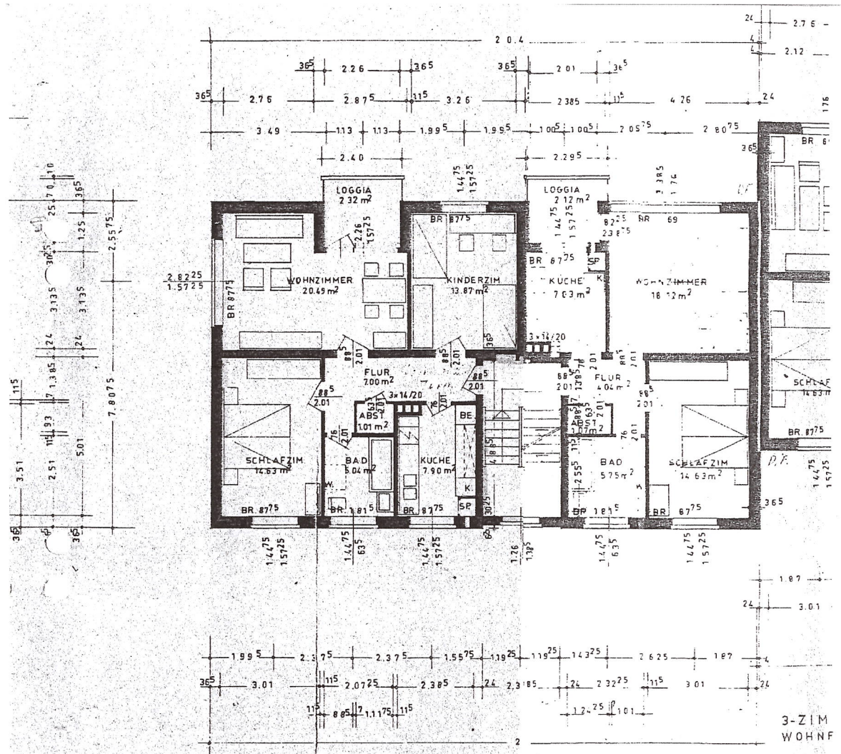
3-ZIMMER-WOHNF WOHNFLÄCHE: 72.26 m 2
