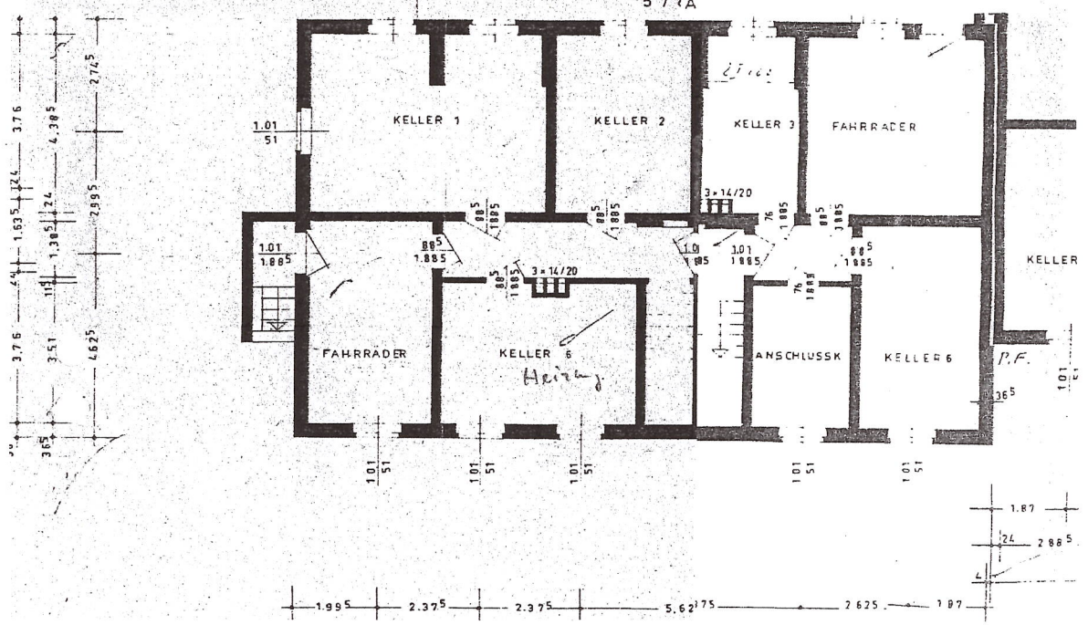
Grundriss KG und Wohnetage
