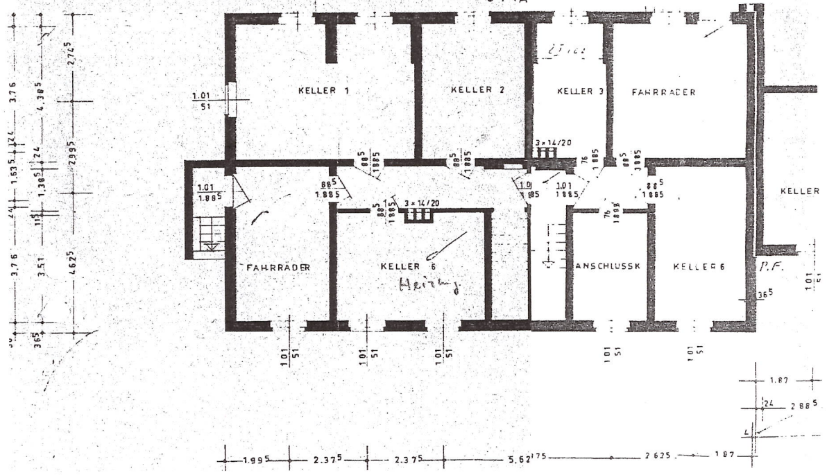
Grundriss KG und Wohntage
