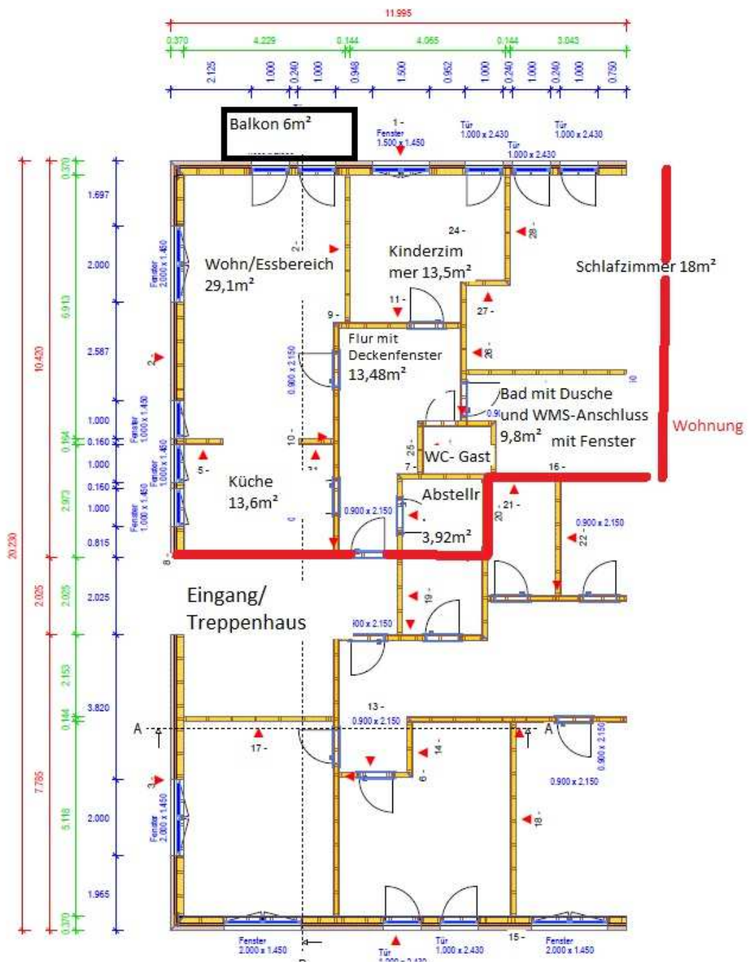
Grundriss Objekt 10649
