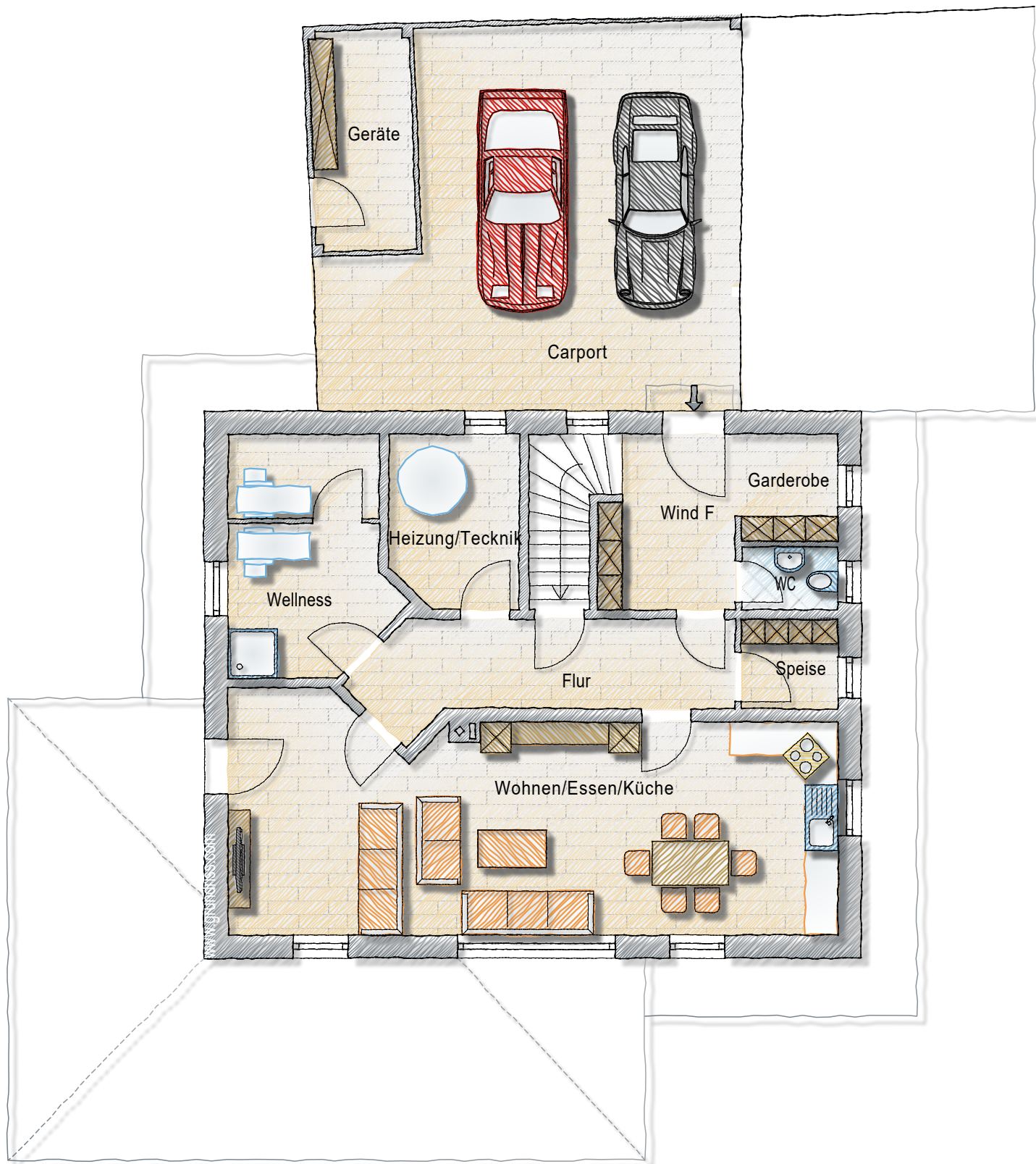
Erdgeschoss
