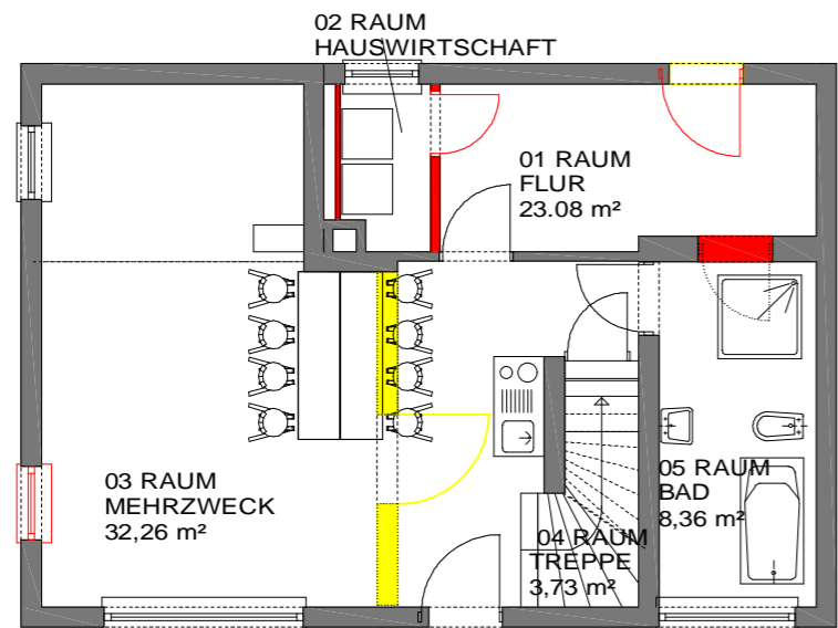
GRUNDRISS ERDGESCHOSS
