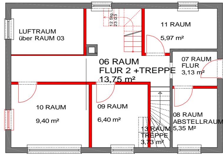
GRUNDRISS 1.OBERGESCHOSS
