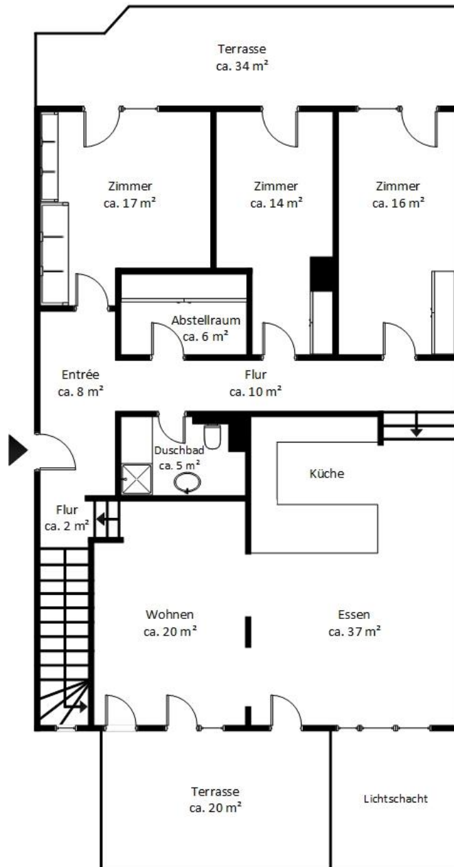
Erdgeschoss
