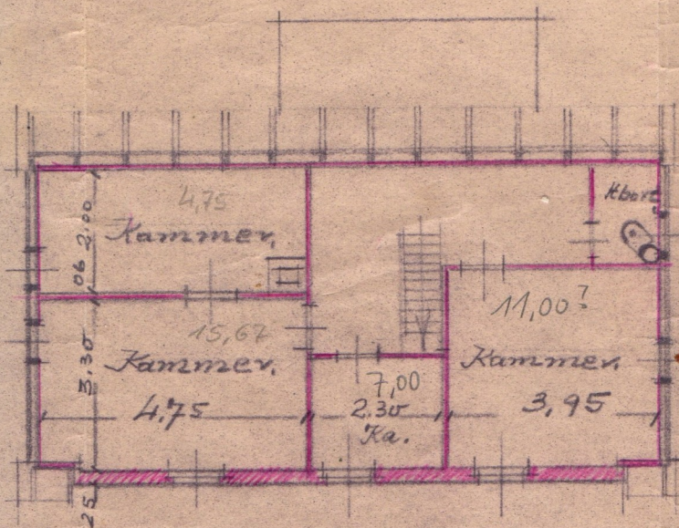
Dachgeschoss.
