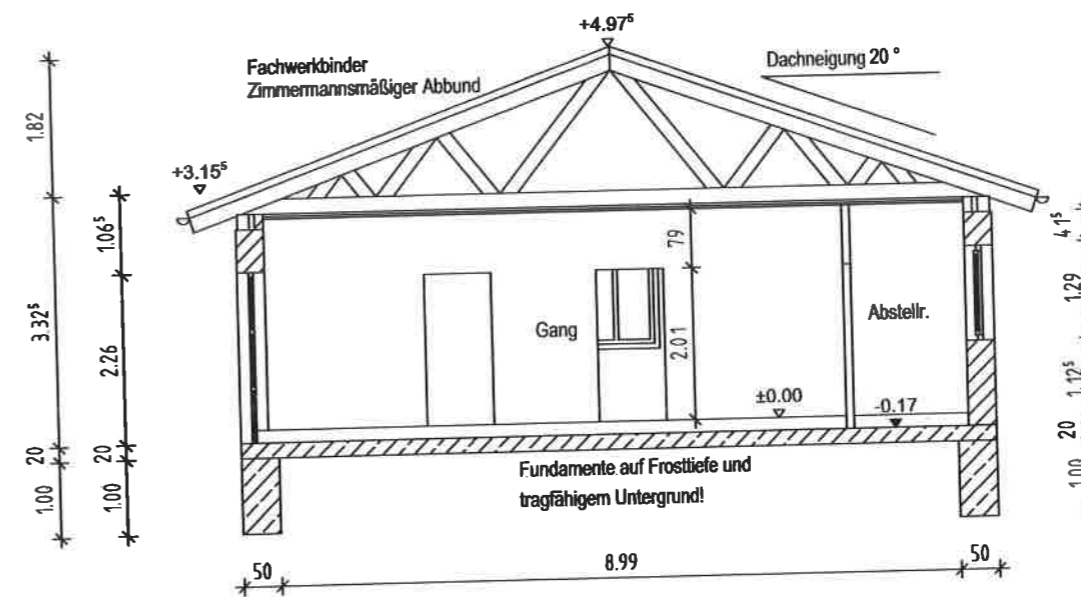
Schnitt A-A
