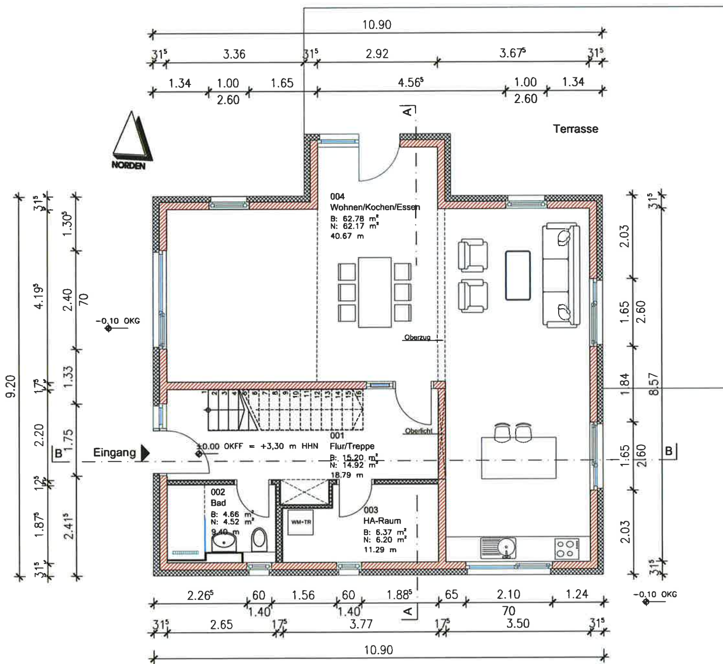
Erdgeschoss Grundriss
