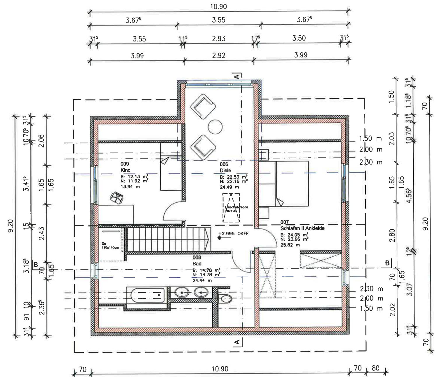
Dachgeschoss Grundriss
