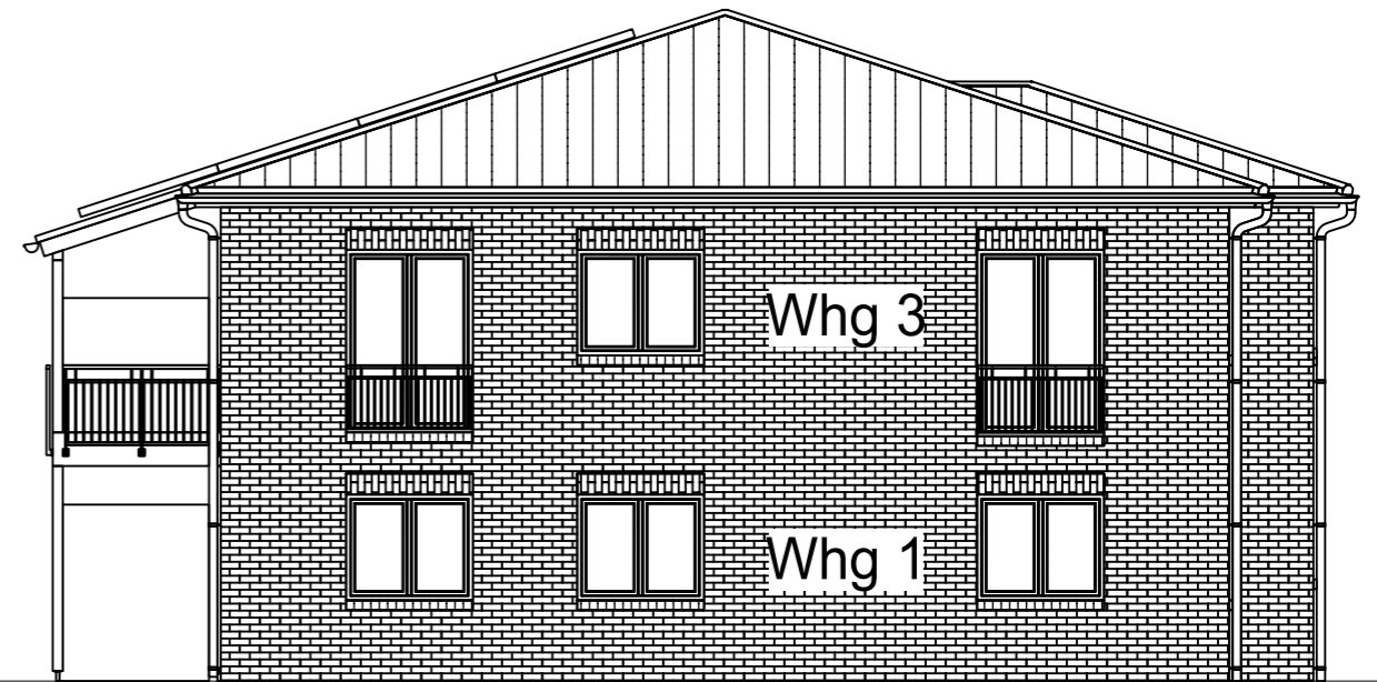
Ansicht Osten
