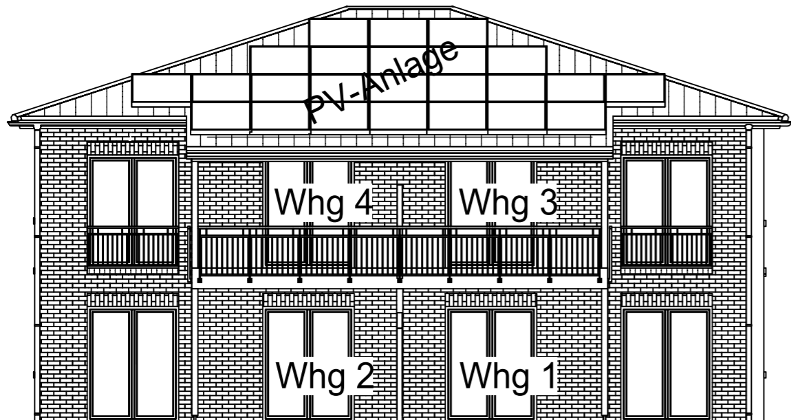
Ansicht Süden
