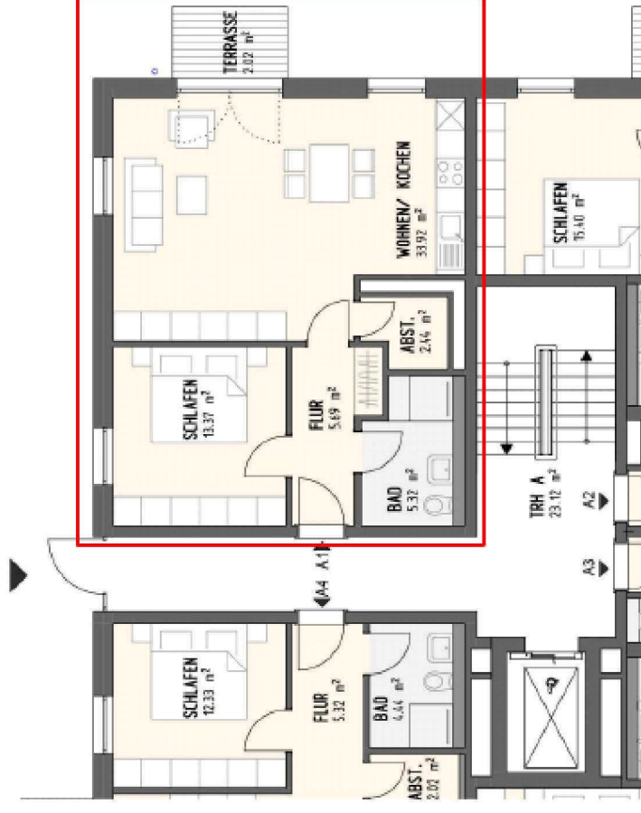
WOHNUNG A1 (2 ZIMMER) M 1:100
