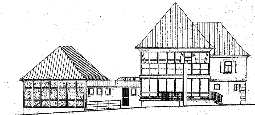
NORD – Ansicht Wohnhaus mit Schwimmhalle u. Wintergarten
