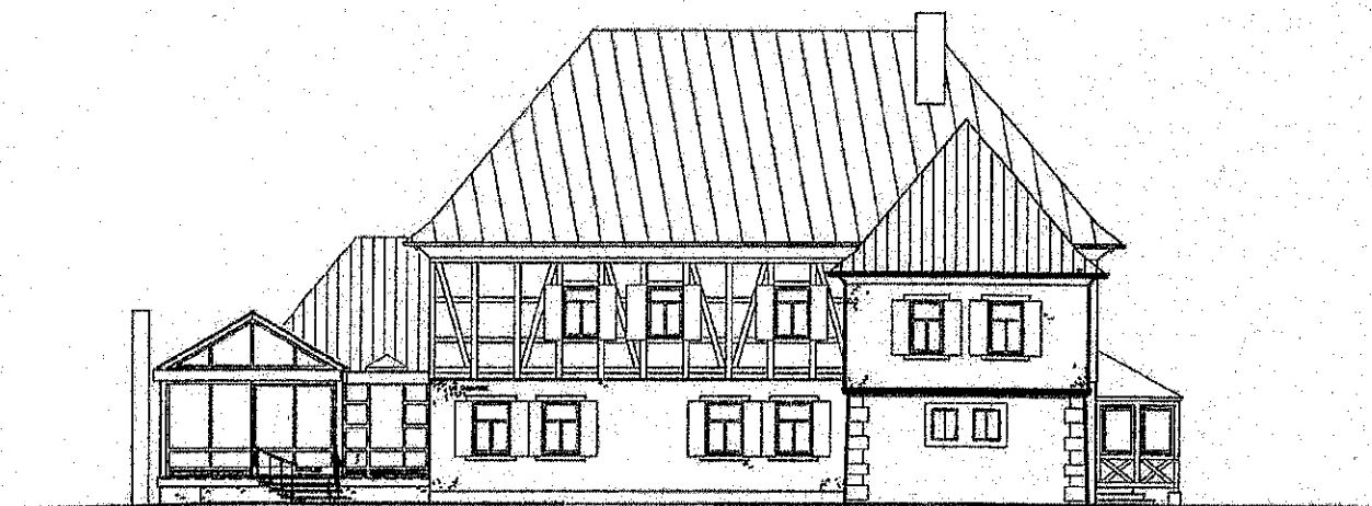
WEST – Ansicht Wohnhaus mit Wintergarten
