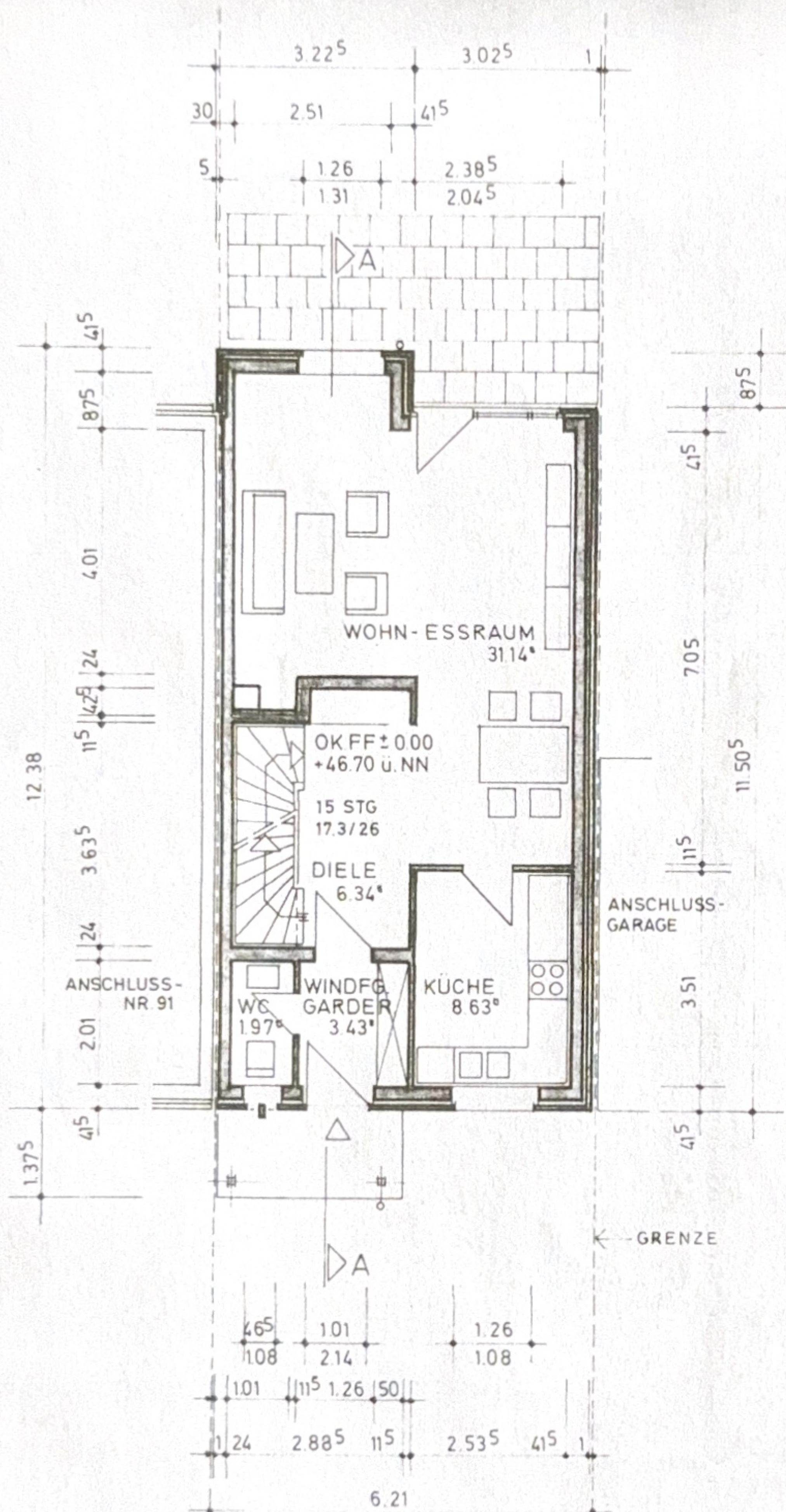
ERDGESCHOSS
